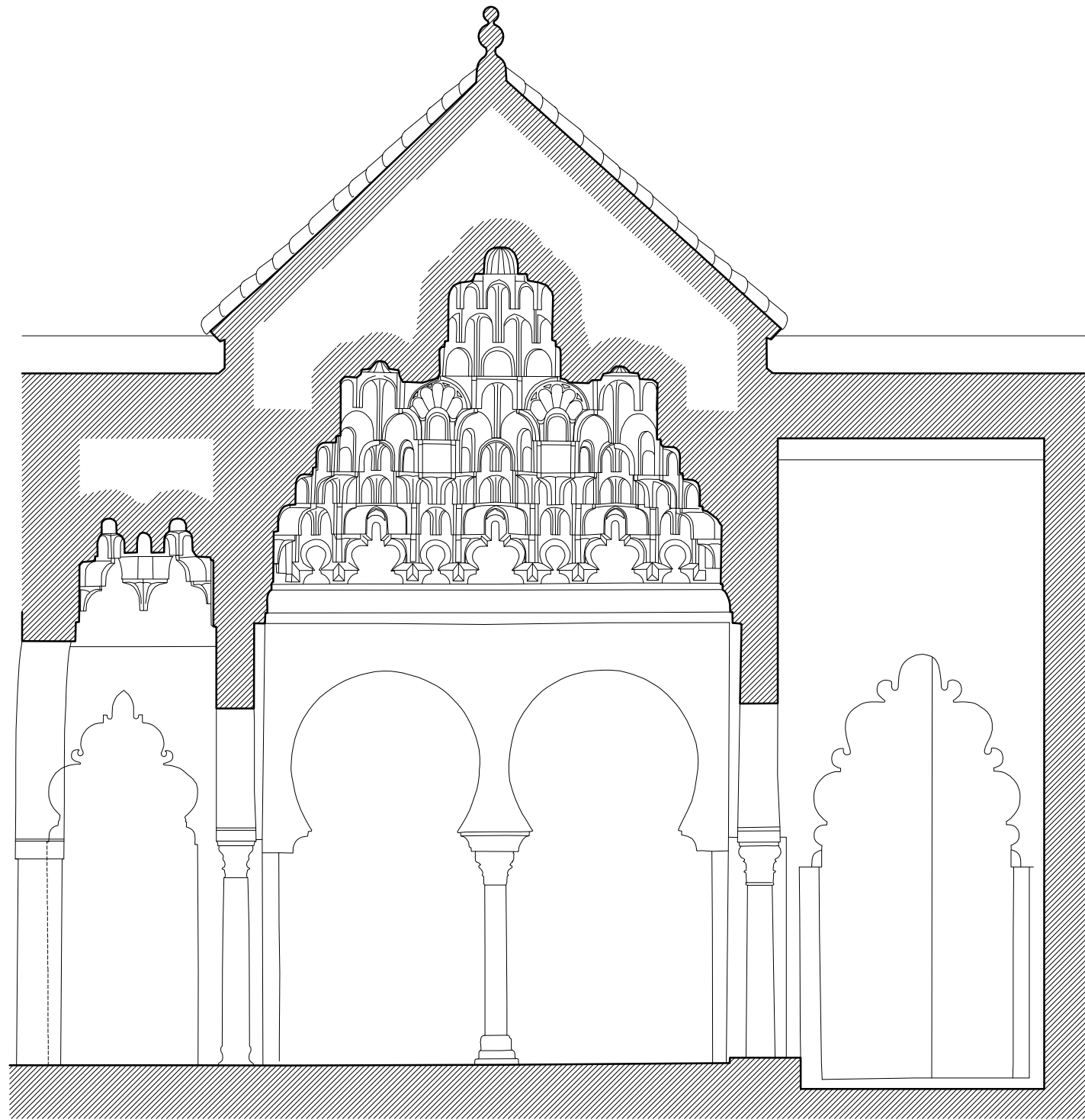
MEZQUITA AL-QARAWIYYIN DE FEZ. MEZQUITA DE LOS MUERTOS. SECCIONES
