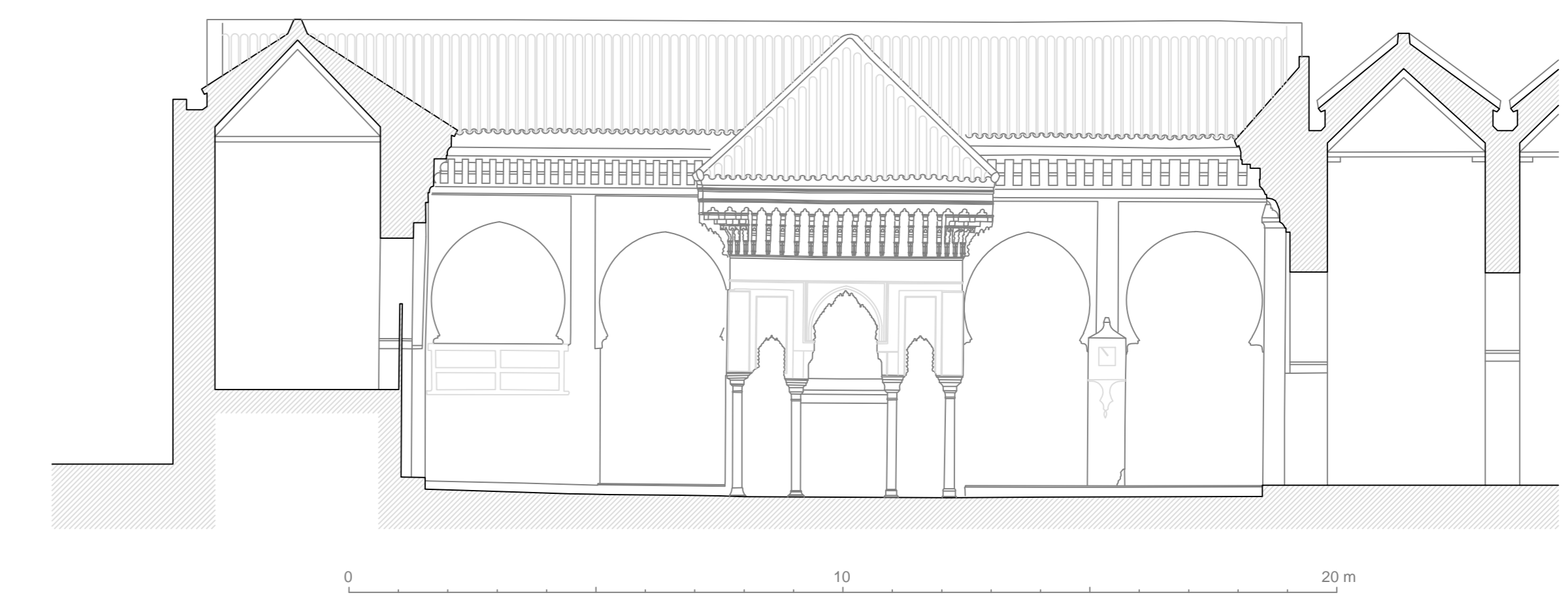
MEZQUITA DE AL-QARAWIYYIN (FEZ). Alzado Este ESQUELA DE ESTUDIOS ARABES. C.S.I.C. junio 2018. A.ALMAGRO e I. ALMELA
