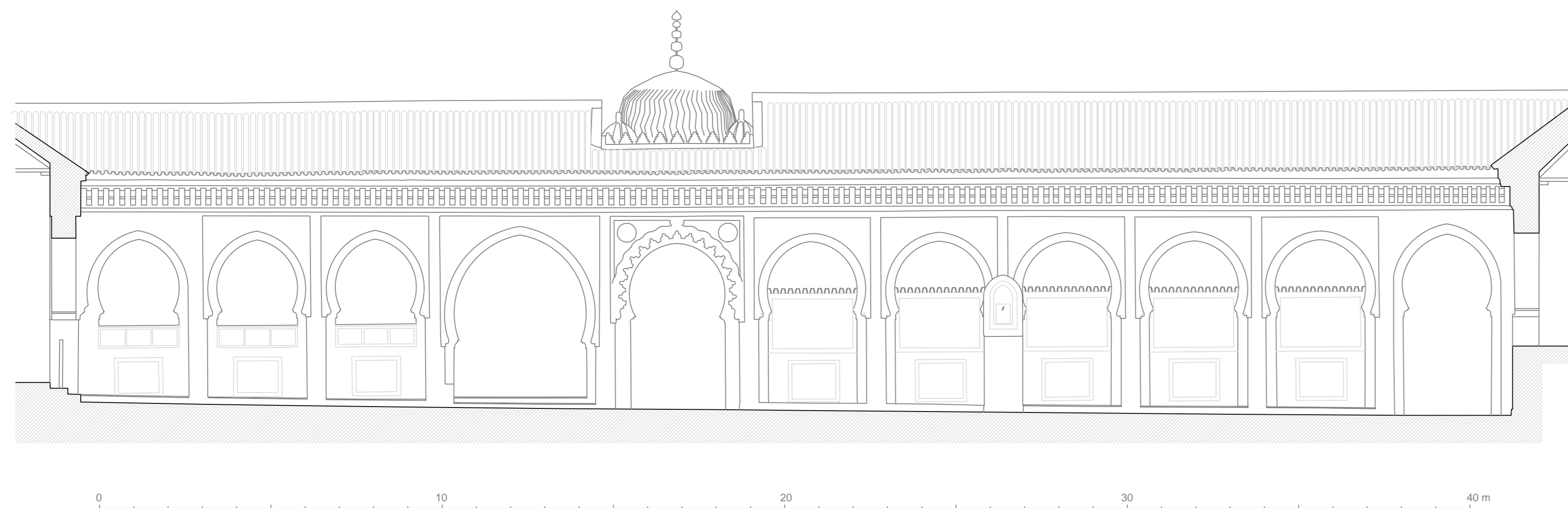
MEZQUITA DE AL-QARAWIYYIN (FEZ). Alzado Norte ESQUELA DE ESTUDIOS ARABES. C.S.I.C. junio 2018. A.ALMAGRO e I. ALMELA
