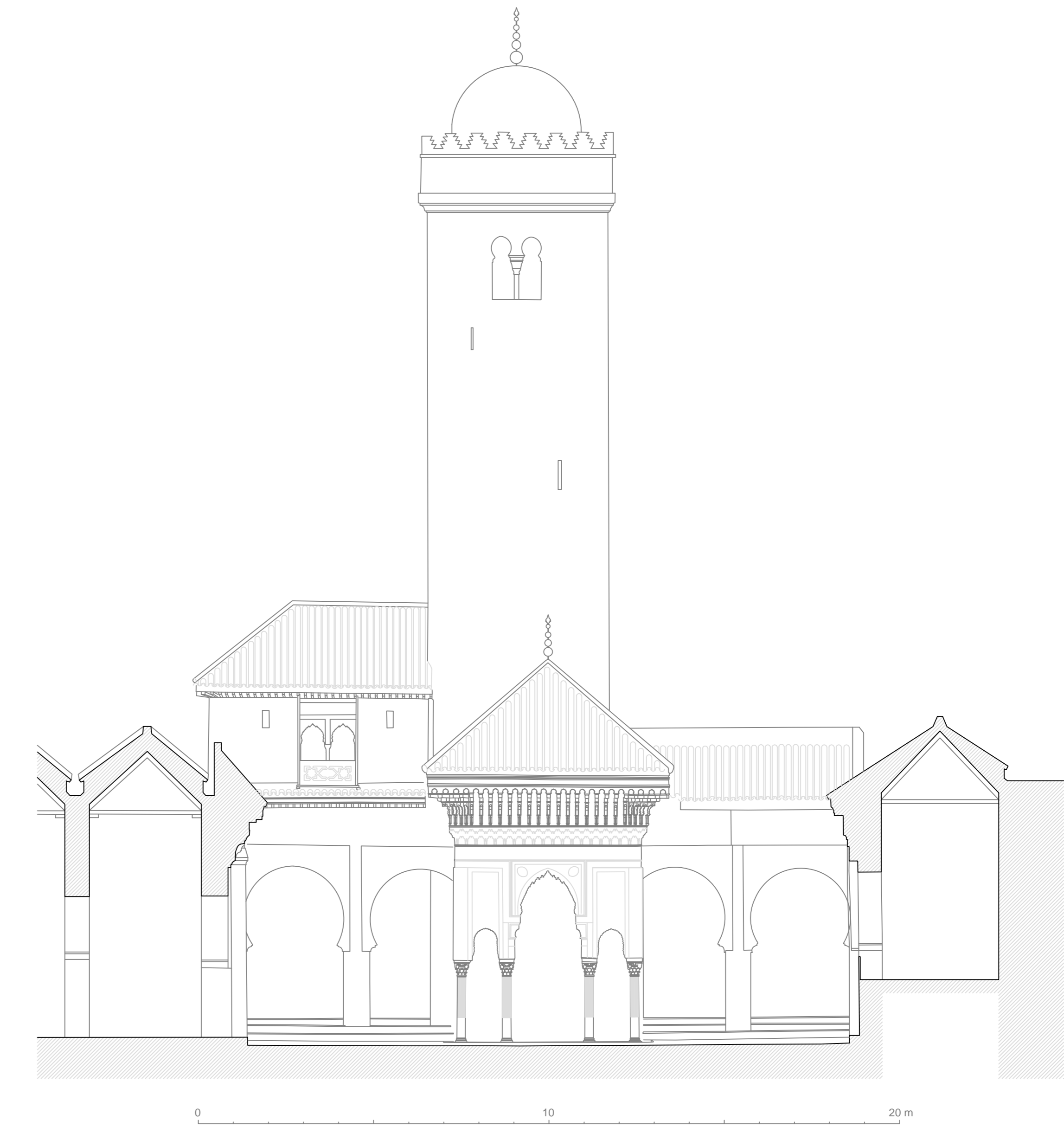
MEZQUITA DE AL-QARAWIYYIN (FEZ). Alzado Oeste ESQUELA DE ESTUDIOS ARABES. C.S.I.C. junio 2018. A.ALMAGRO e I. ALMELA
