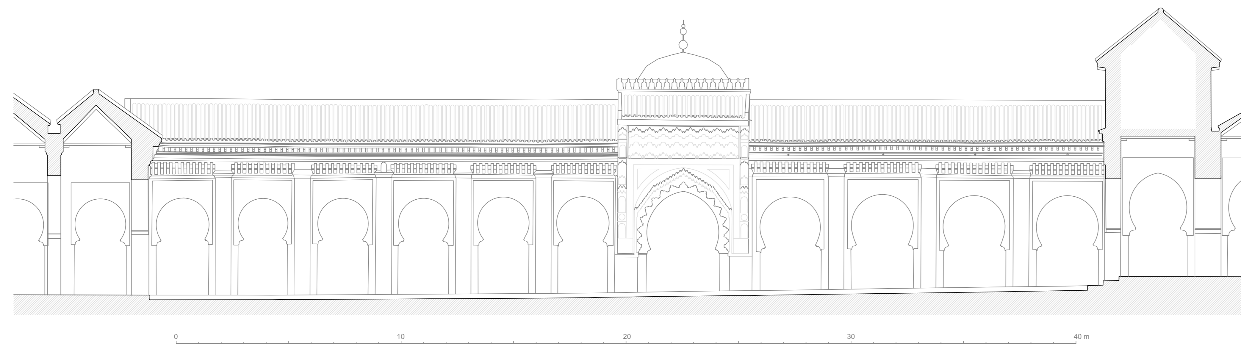
MEZQUITA DE AL-QARAWIYYIN (FEZ). Alzado Sur ESQUELA DE ESTUDIOS ARABES. C.S.I.C. junio 2018. A.ALMAGRO e I. ALMELA
