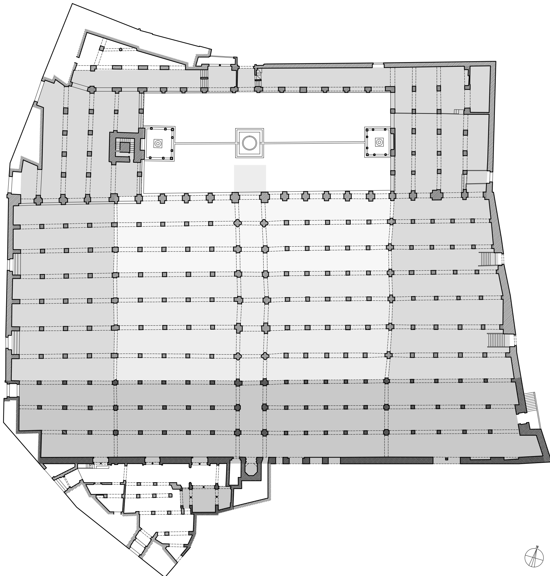
MEZQUITA QARAWIYYIN DE FEZ. PLANTA.
