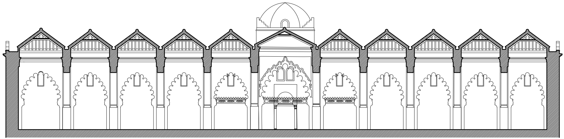
MEZQUITA ALMORÁVIDE DE ARGEL, SECCION TRANSVERSAL POR LA SALA DE ORACION A. ALMAGRO /ARQ. marzo 2017
