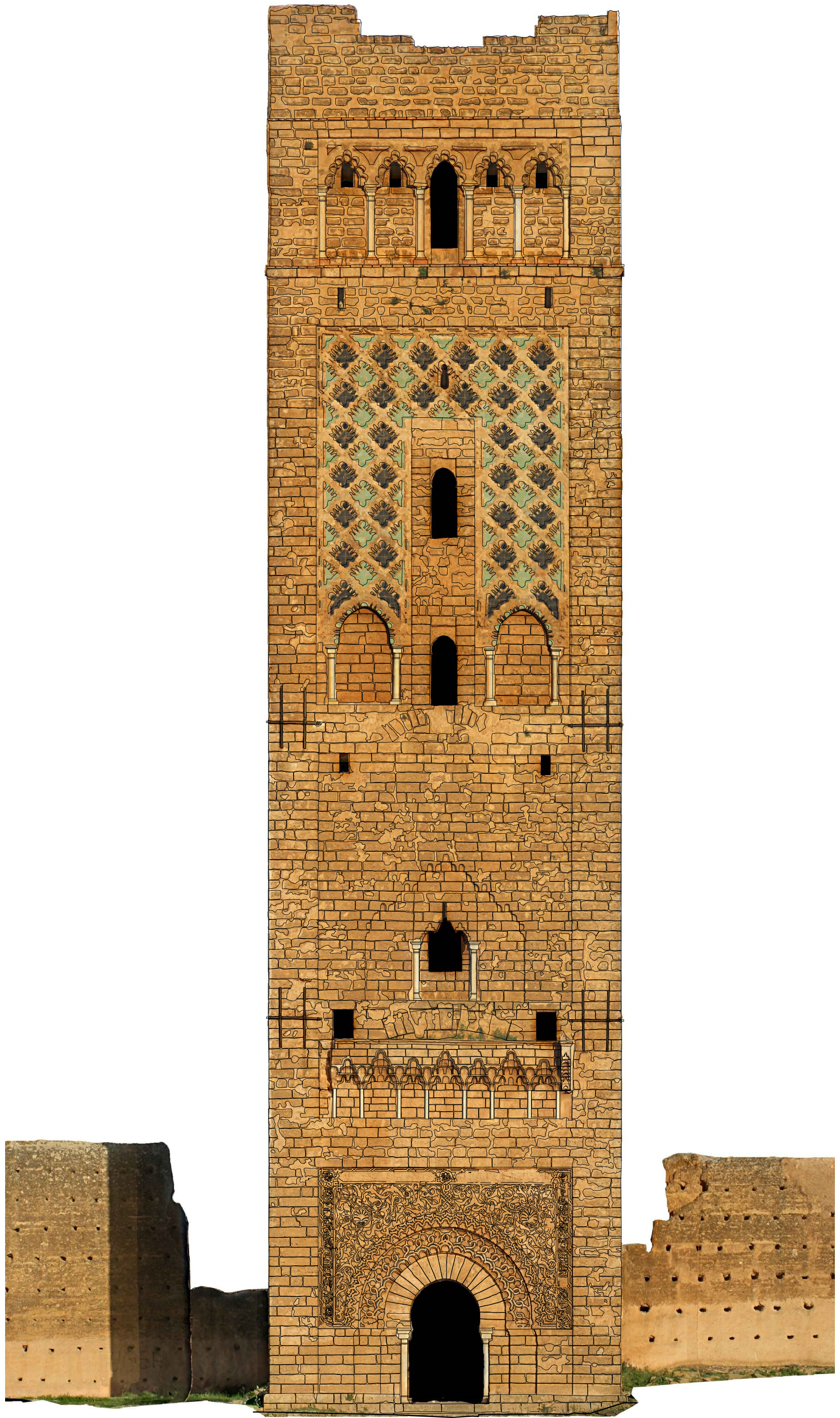
ALMINAR DE LA MEZQUITA DE MANSURA. TREMECÉN (ARGELIA) A. ALMAGRO / arq. S. MORENA / ing. ALZADO N.º.
