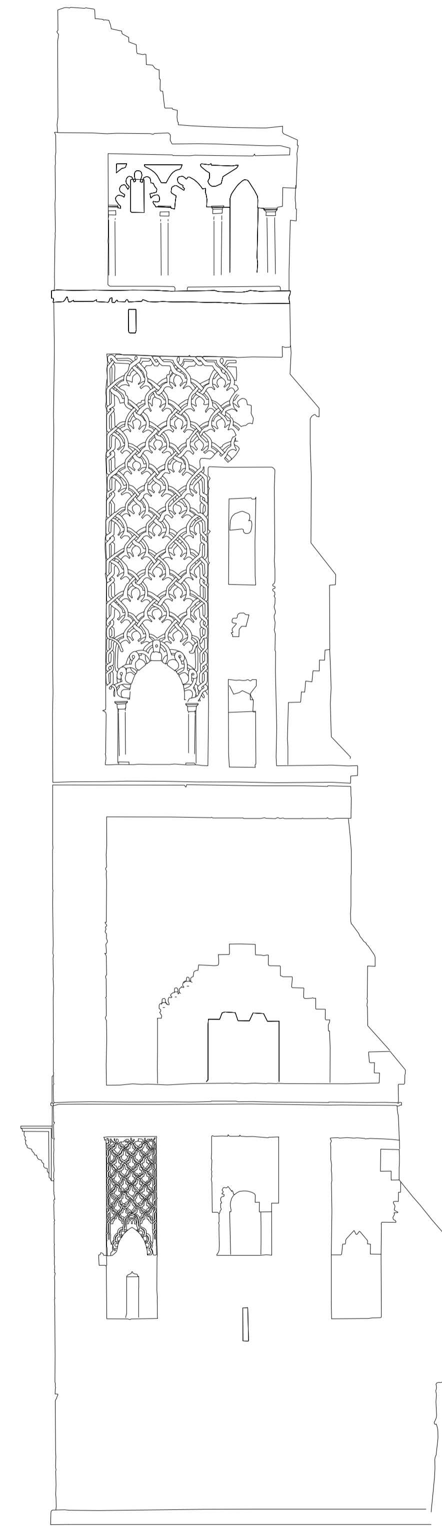
ALMINAR DE LA MEZQUITA DE MANSURA. TREMECÉN (ARGELIA) A. ALMAGRO / arq. S. MORENA / ing. ALZADOS
