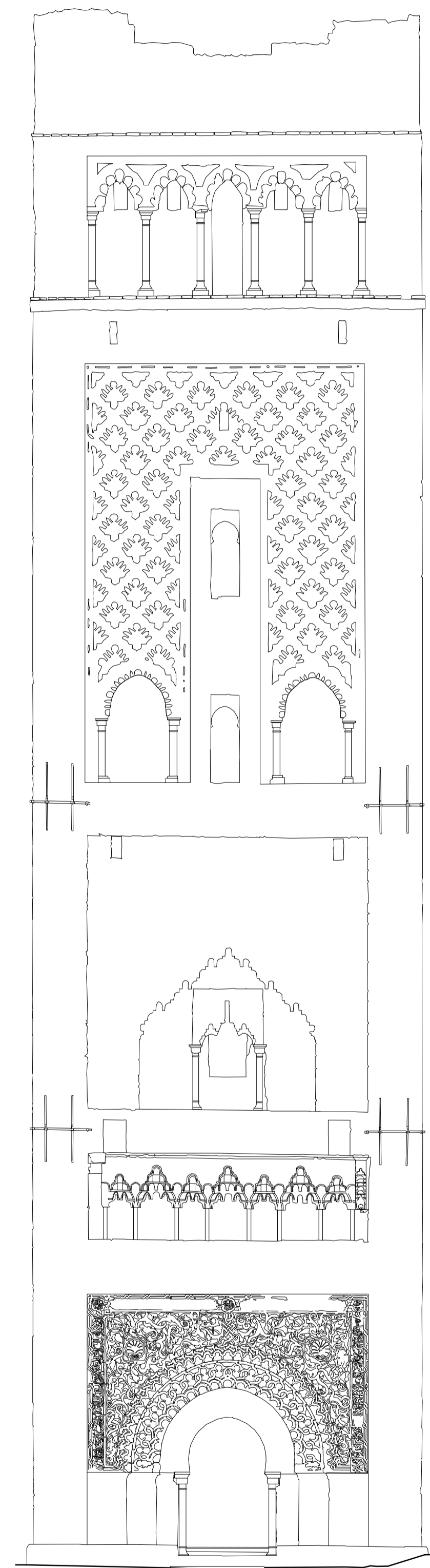
ALMINAR DE LA MEZQUITA DE MANSURA. TREMECÉN (ARGELIA) A. ALMAGRO / arq. S. MORENA / ing. ALZADOS
