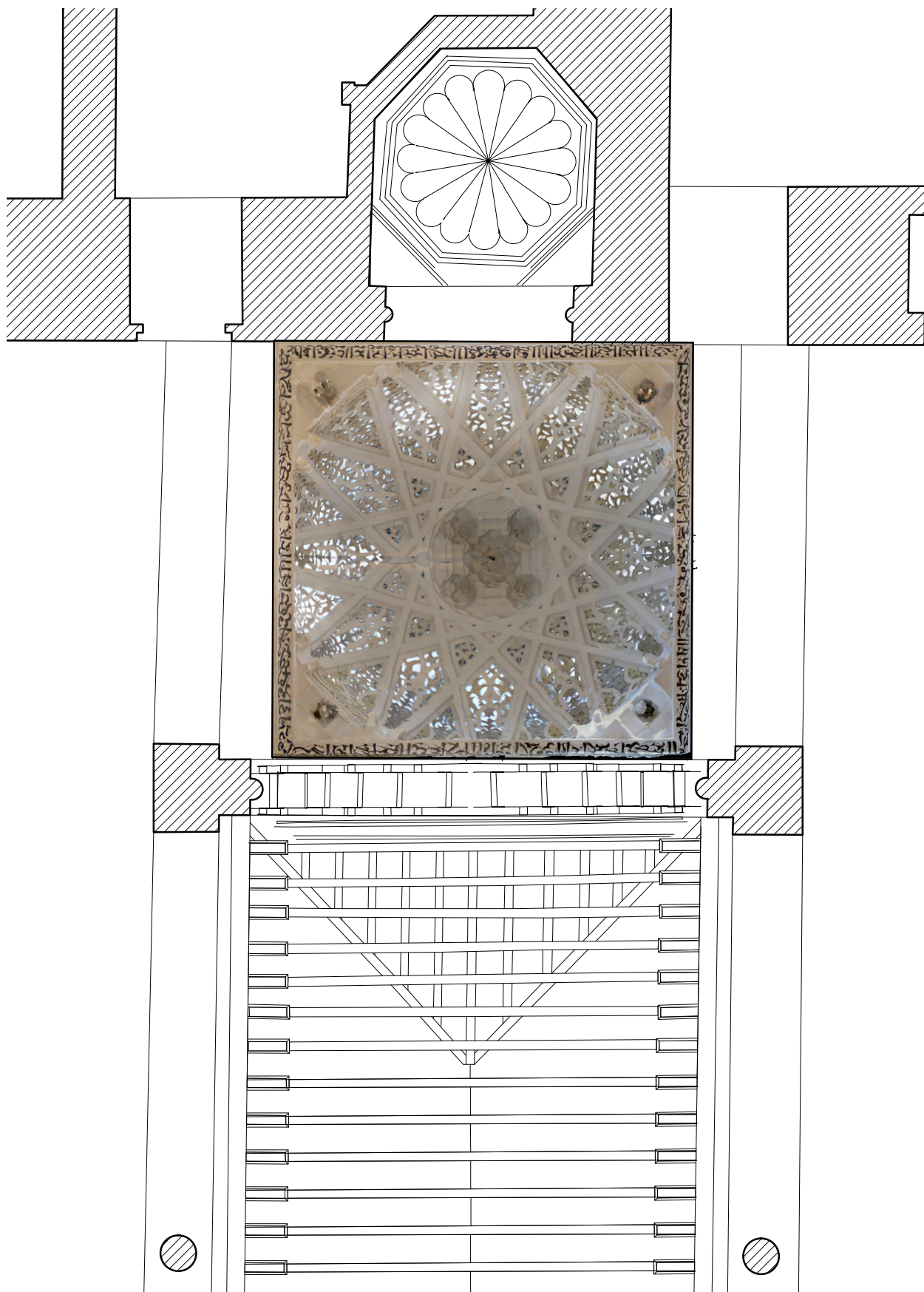
0 1 2 3m MEZQUITA ALMORÁVIDE DE TREMECÉN. MIHRAB Y CÚPULA. A. ALMAGRO /ARQ. OCTUBRE 2011
