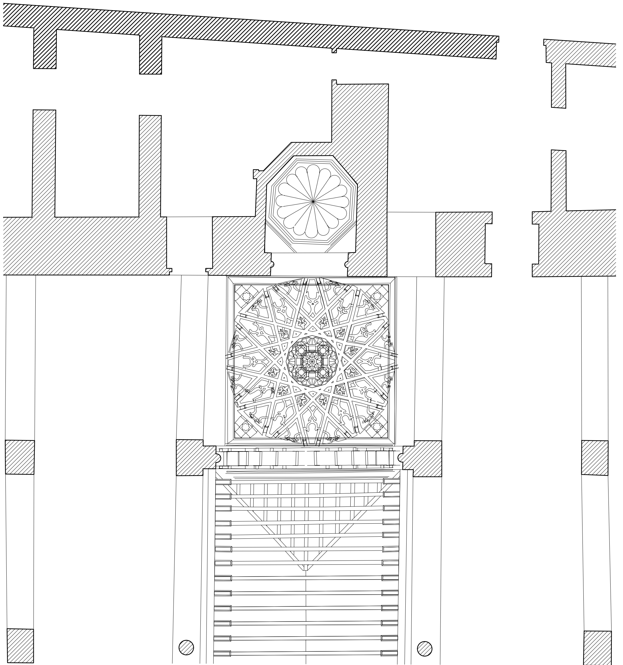
0 1 2 3 m MEZQUITA ALMORÁVIDE DE TREMECÉN. MIHRAB Y CÚPULA. A. ALMAGRO /ARQ. OCTUBRE 2011
