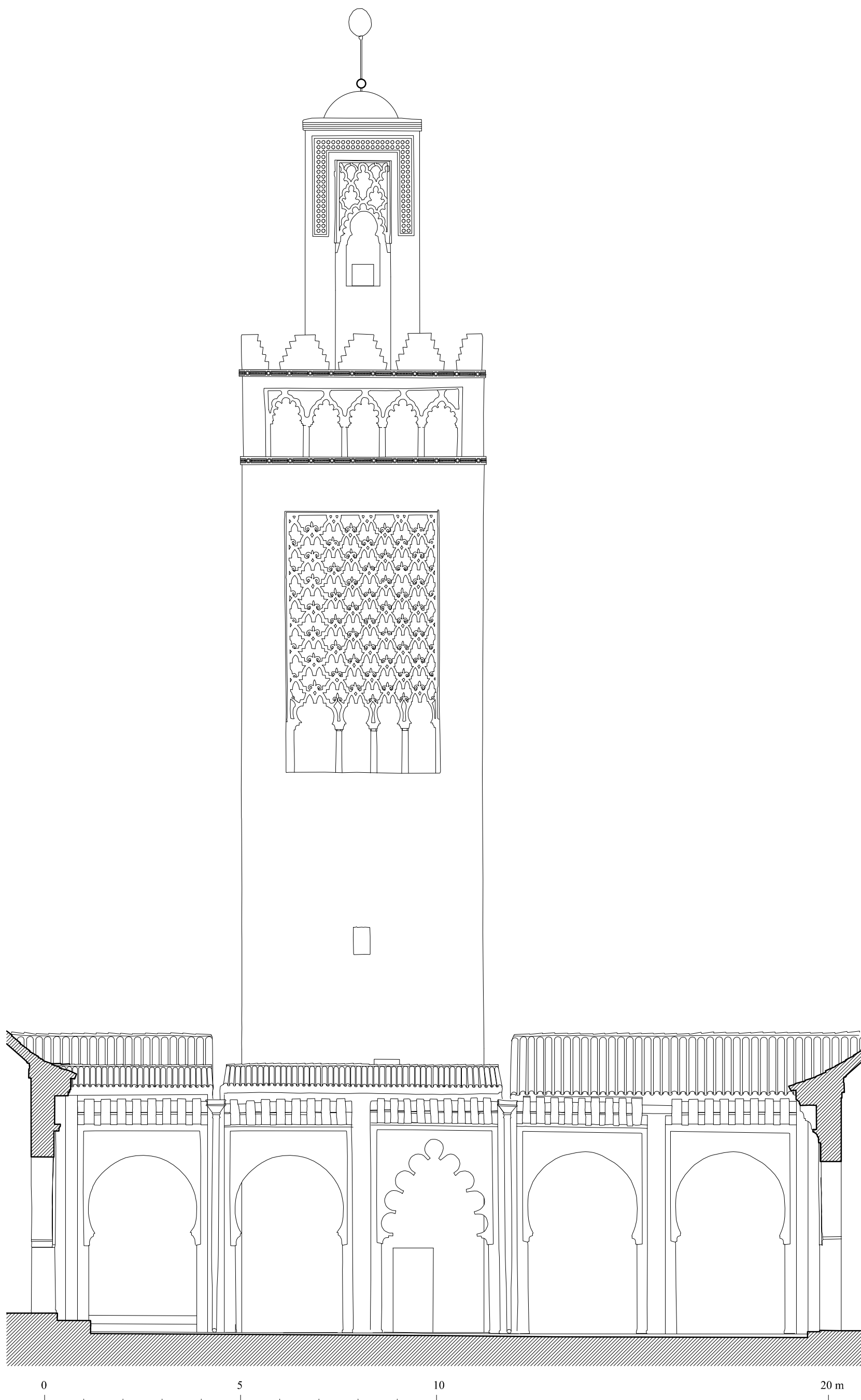
GRANDE MOSQUÉE DE TLEMCEEN. ELEVATION SUD DU MINARET A.ALMAGRO, arch. (EEA, CSIC)
