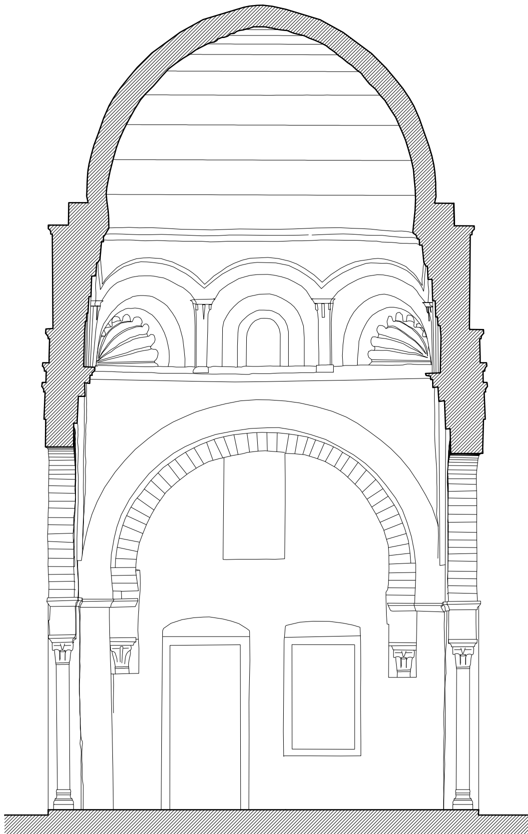
0 1 2 3 m MAUSOLEE DE SIDI BOUKHRISANE RESTITUTION PHOTOGRAMMETRIQUE. ESCUELA DE ESTUDIOS ARABES. GRANADA.
