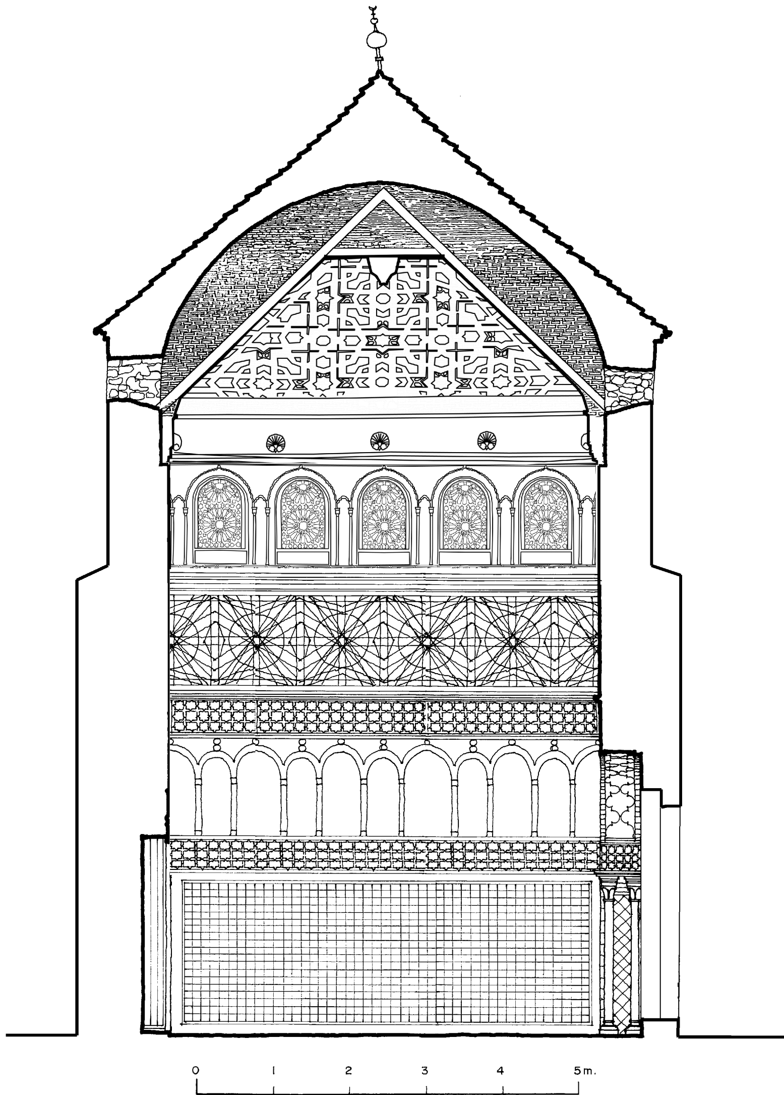
ZAWIYA DE SIDI QASIM AL-ZALIJI. TUNEZ. SECCION DEL MAUSOLEO HIPÓTESIS
