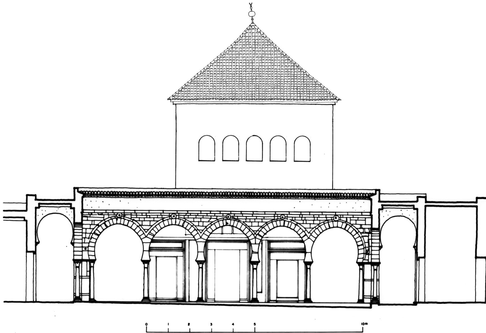
ZAWIYA DE SIDI QASIM AL-ZALIJI. TUNEZ. ALZADO HIPOTETICO s. XVI
