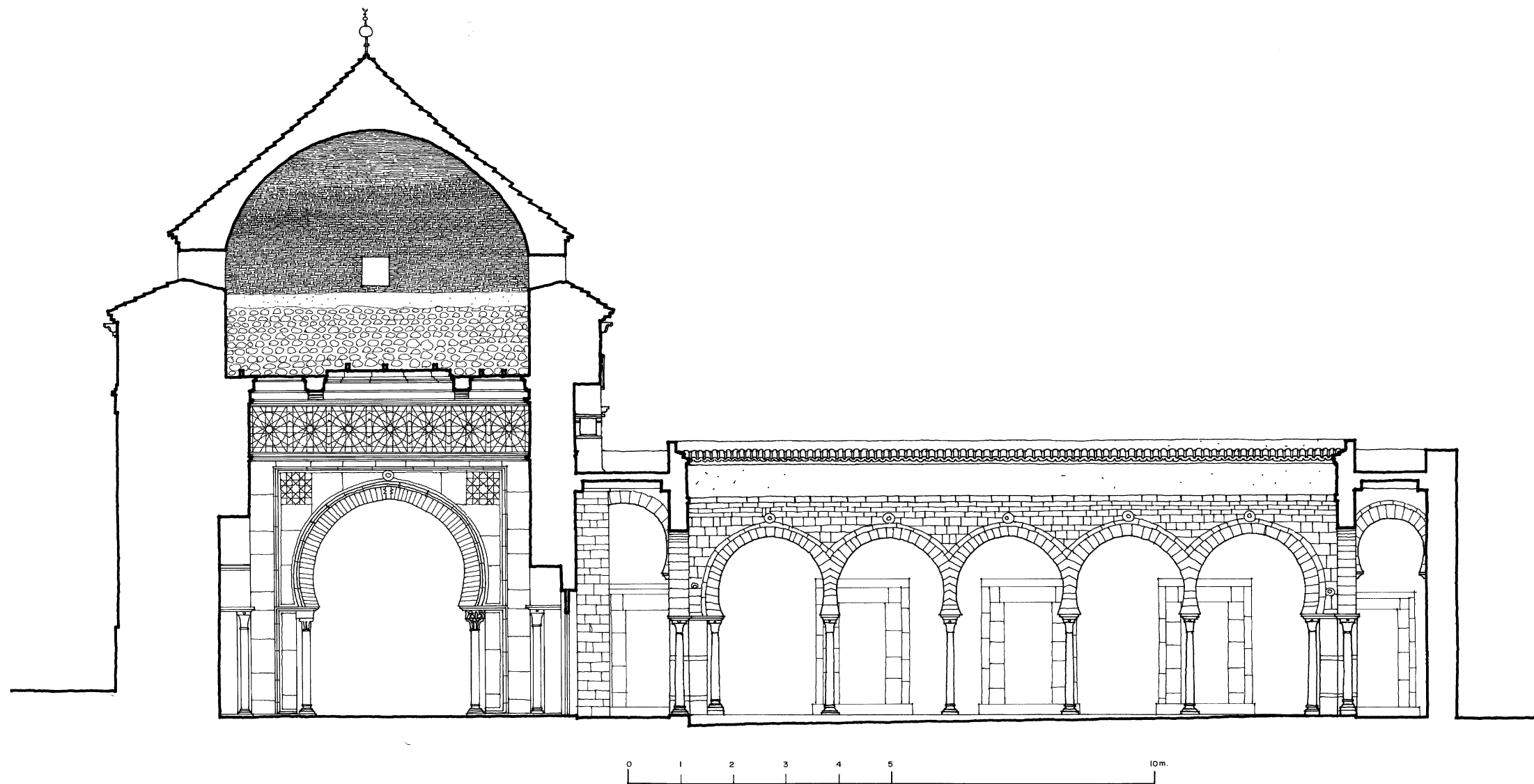
ZAWIYA DE SIDI QASIM AL-ZALIJI. TUNEZ. SECCION TRANSVERSAL DEL MAUSOLEO Y EL PATIO
