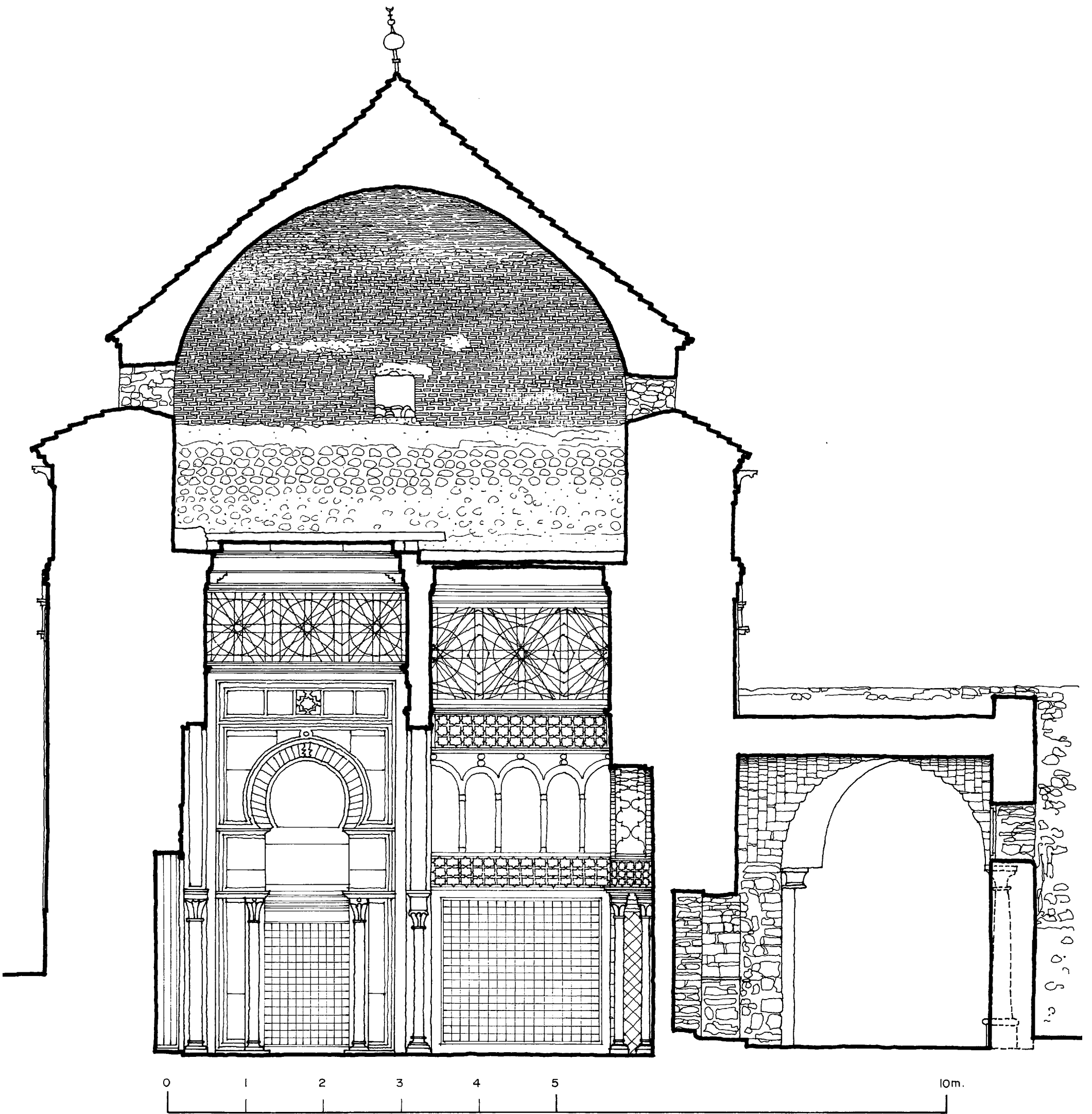
ZAWIYA DE SIDI QASIM AL-ZALIJI. TUNEZ. SECCION N-S DEL MAUSOLEO
