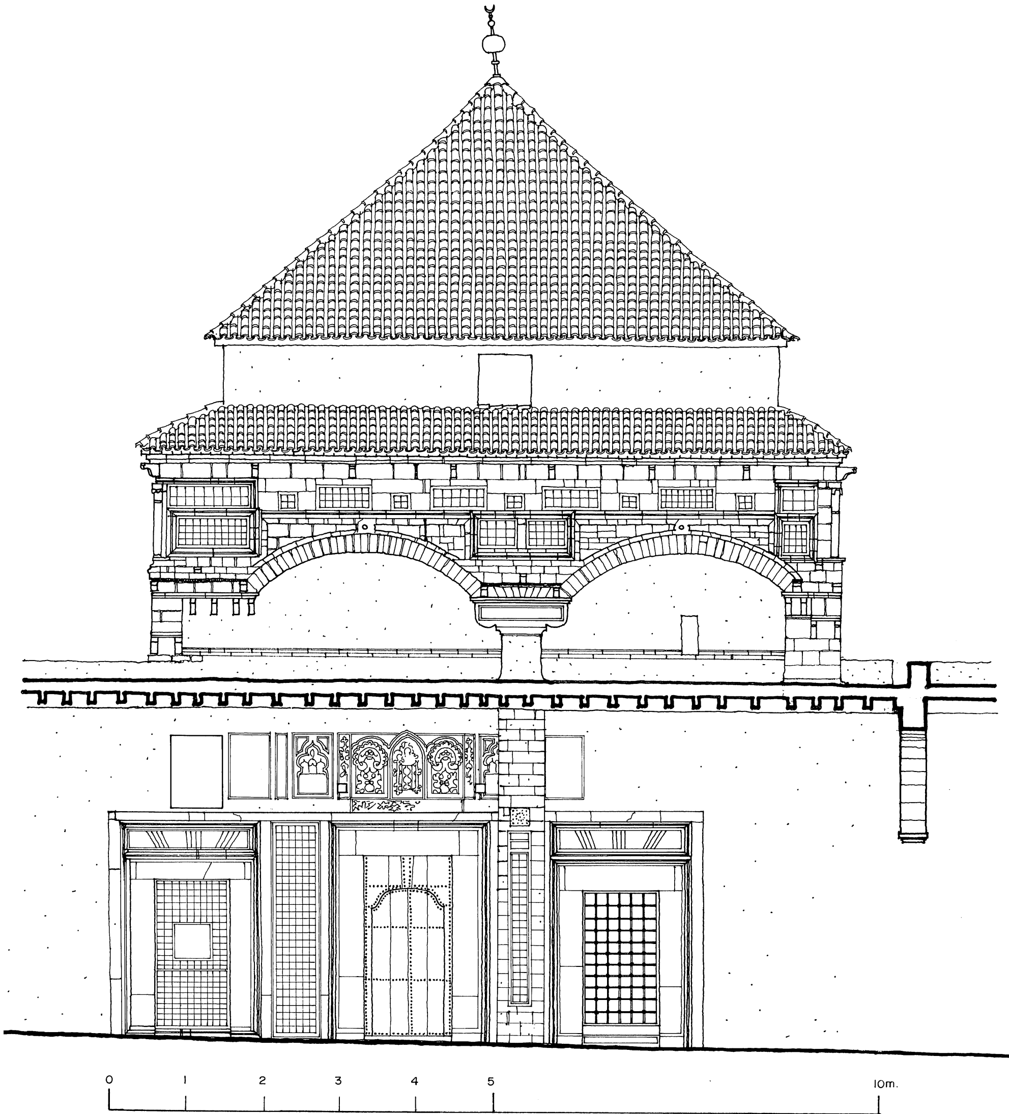
ZAWIYA DE SIDI QASIM AL-ZALIJI. TUNEZ. ALZADO ESTE DEL MAUSOLEO
