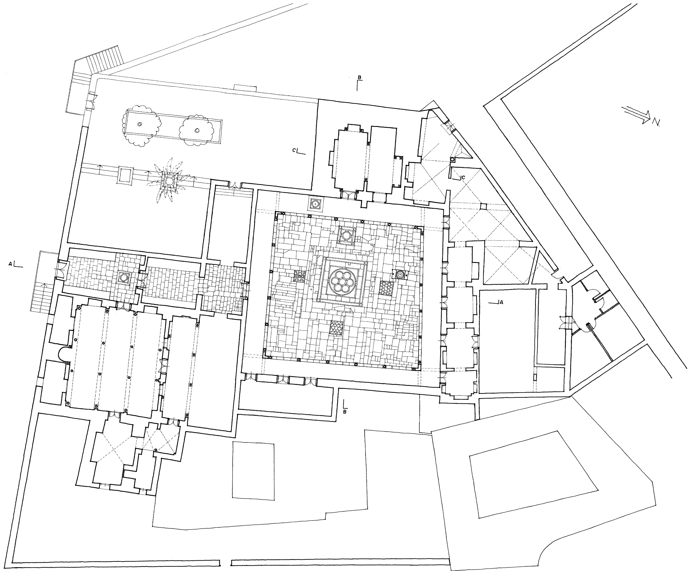
ZAWIYA DE SIDI QASIM AL-ZALIJI. TUNEZ. PLANTA GENERAL FINAL
