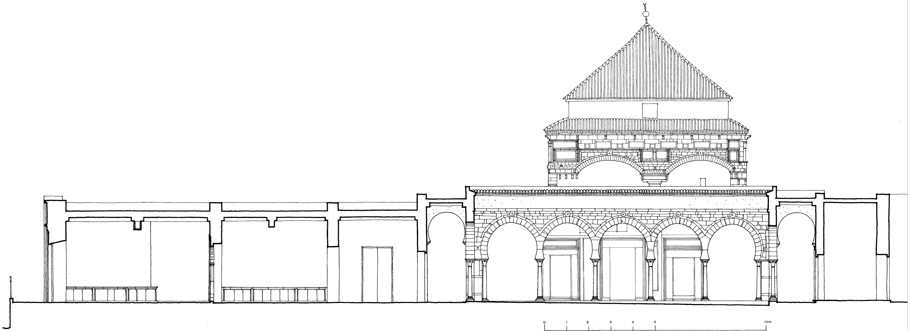
ZAWIYA DE SIDI QASIM AL-ZALIJI. TUNEZ. SECCION LONGITUDINAL
