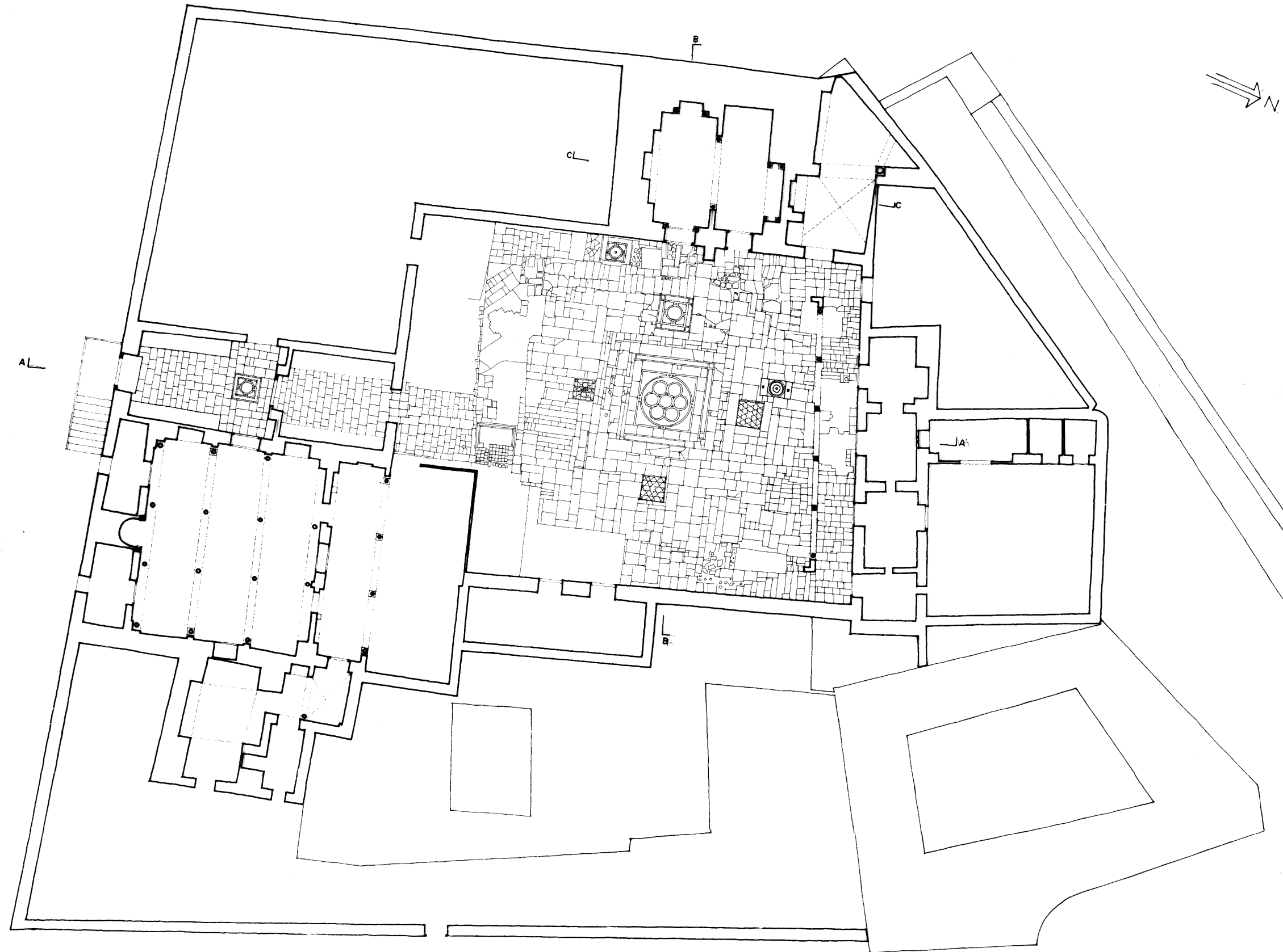
ZAWIYA DE SIDI QASIM AL-ZALIJI. TUNEZ. PLANTA GENERAL INICIAL
