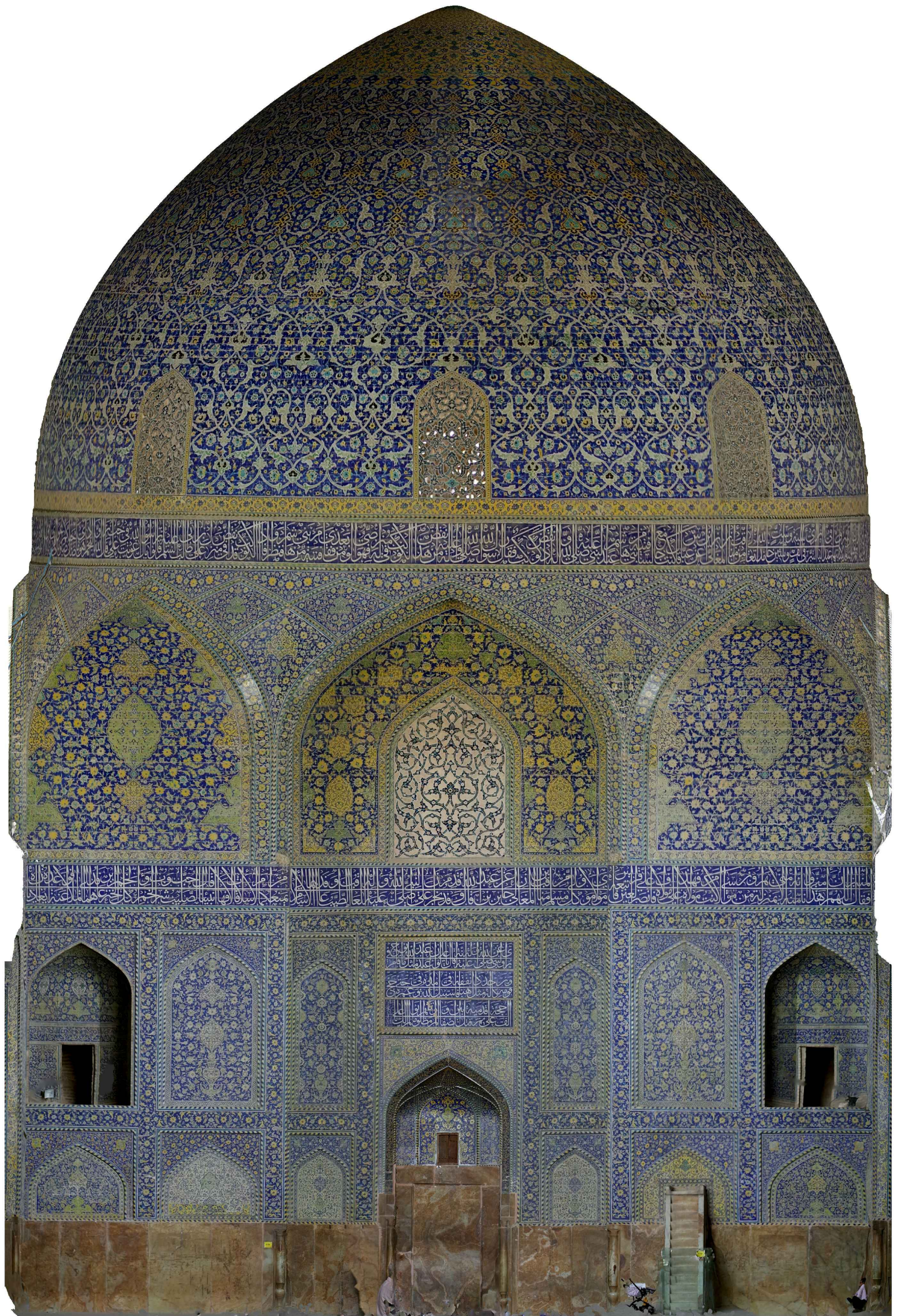
0 5 10 15 20m MASJID-I SAH. ISFAHAN. SALA DE ORACION Y MIHRAB. SECCION A.Almagro / arq. RABASF mayo 2019
