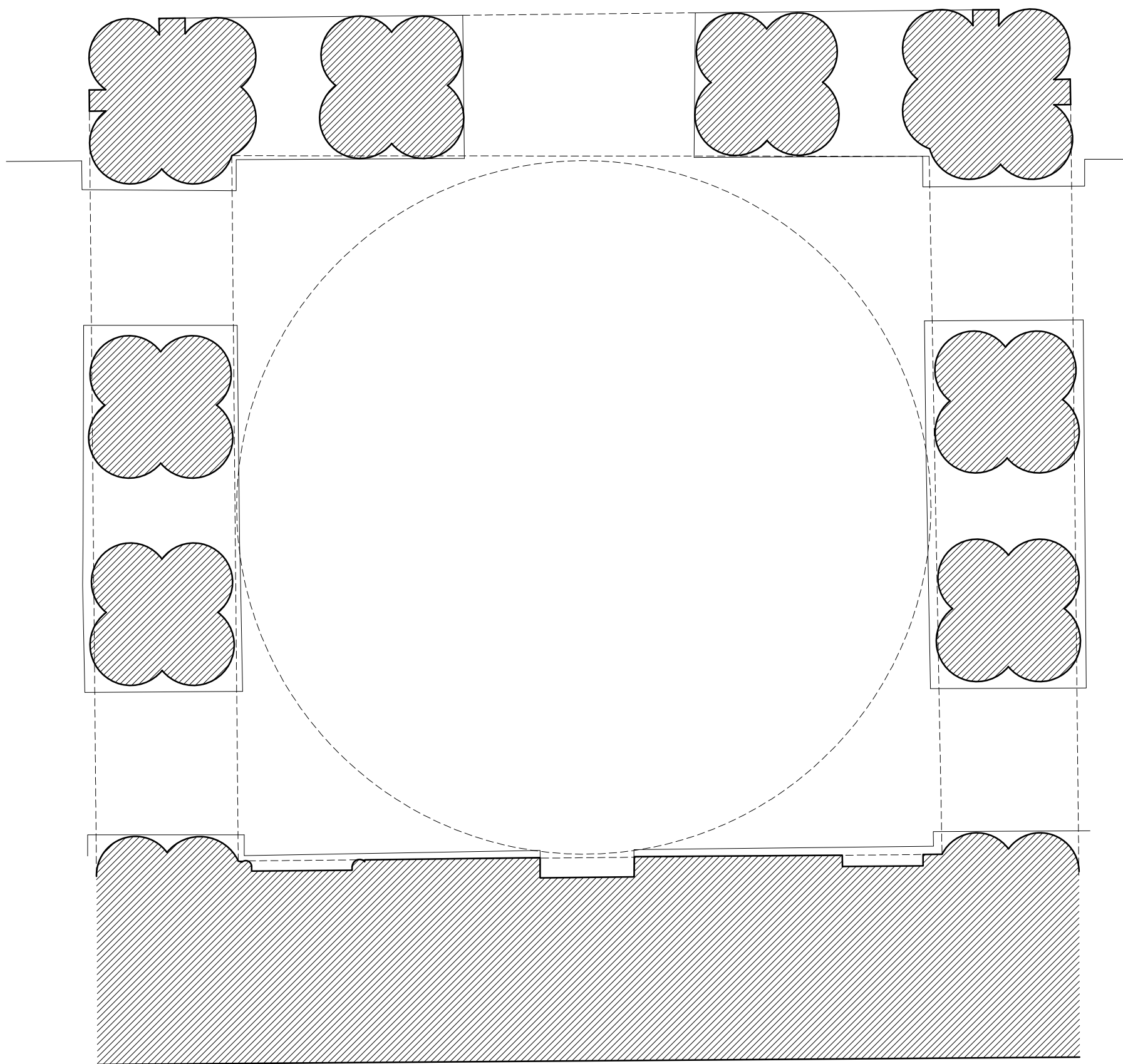
0 5 10 15 20 m MASJID-I-JAMI. ISFAHAN. QUBBA SUR Y MIHRAB. PLANTA A.Almagro / arq. RABASF mayo 2019
