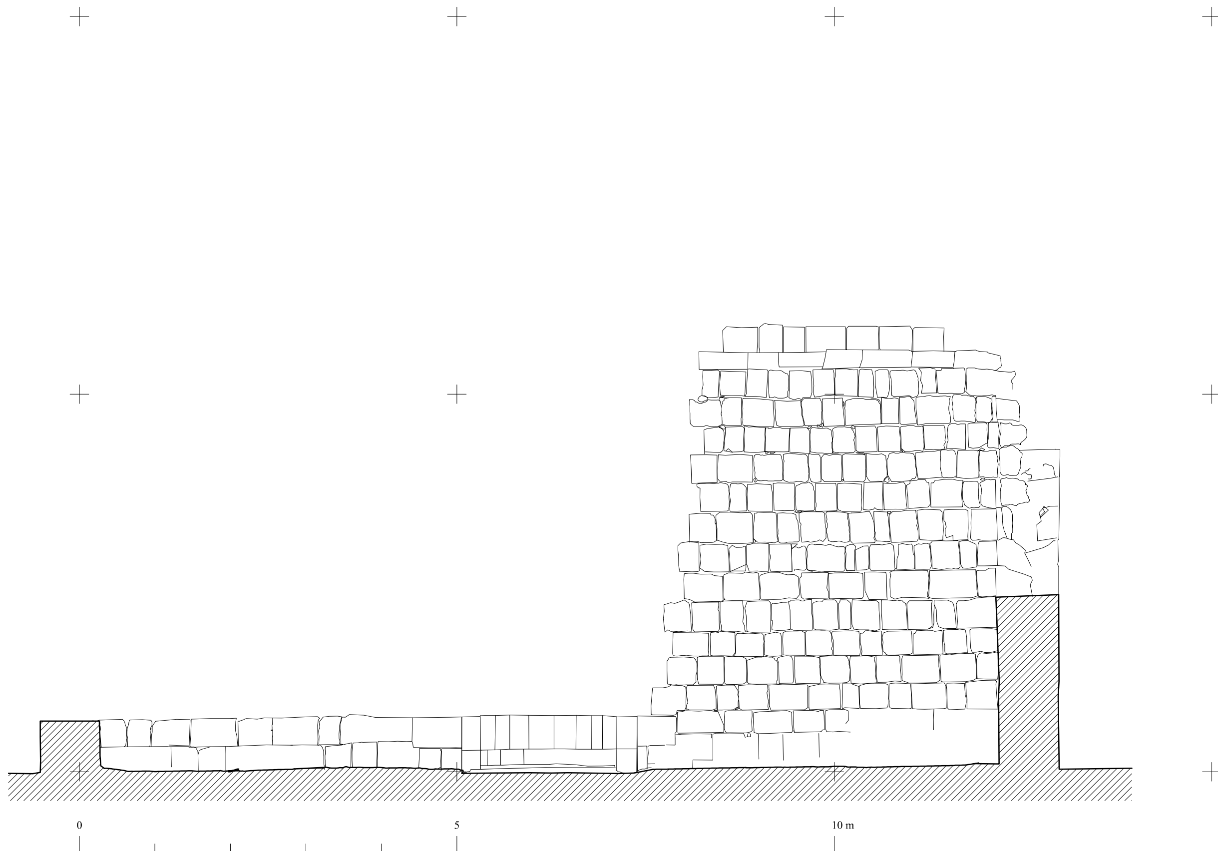
MEZQUITA DE QASR AL-HALLABAT. ALZADO INTERIOR SUR.
