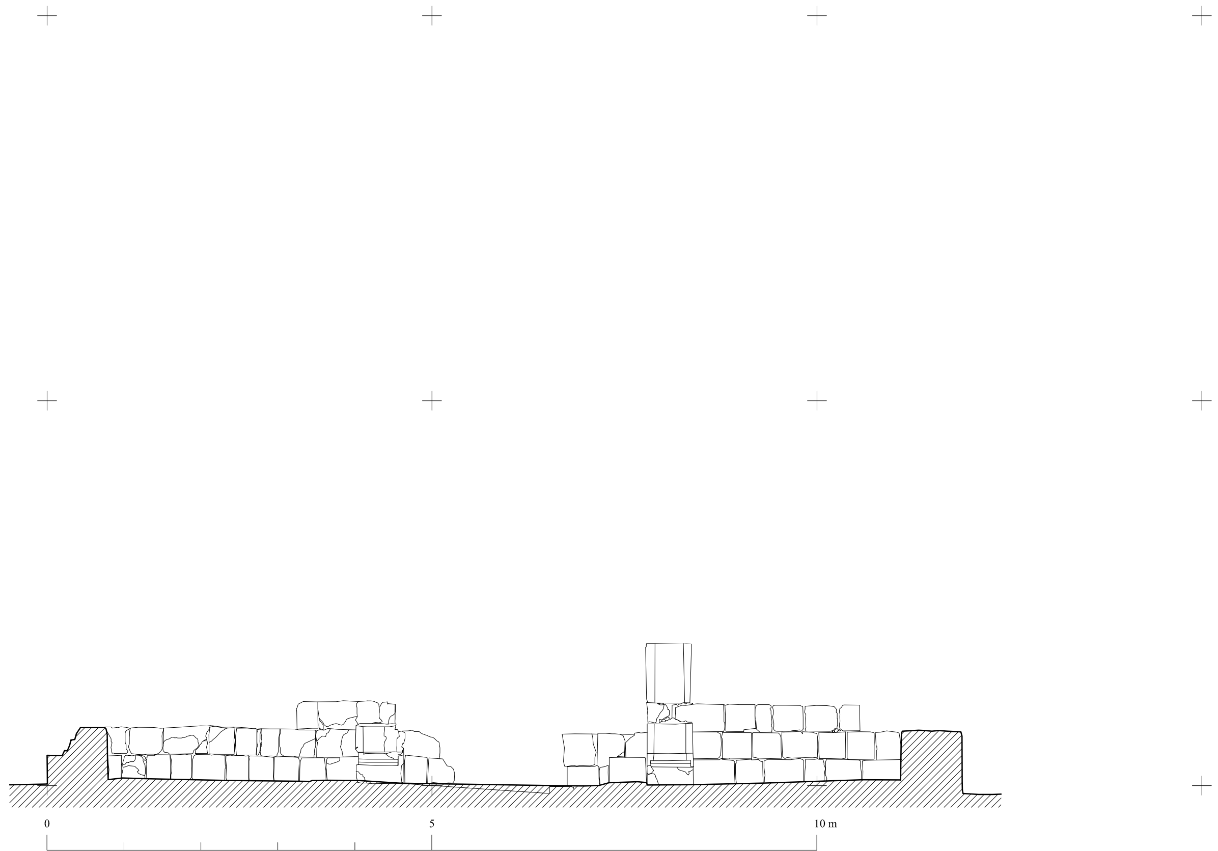
MEZQUITA DE QASR AL-HALLABAT. ALZADO INTERIOR ESTE.
