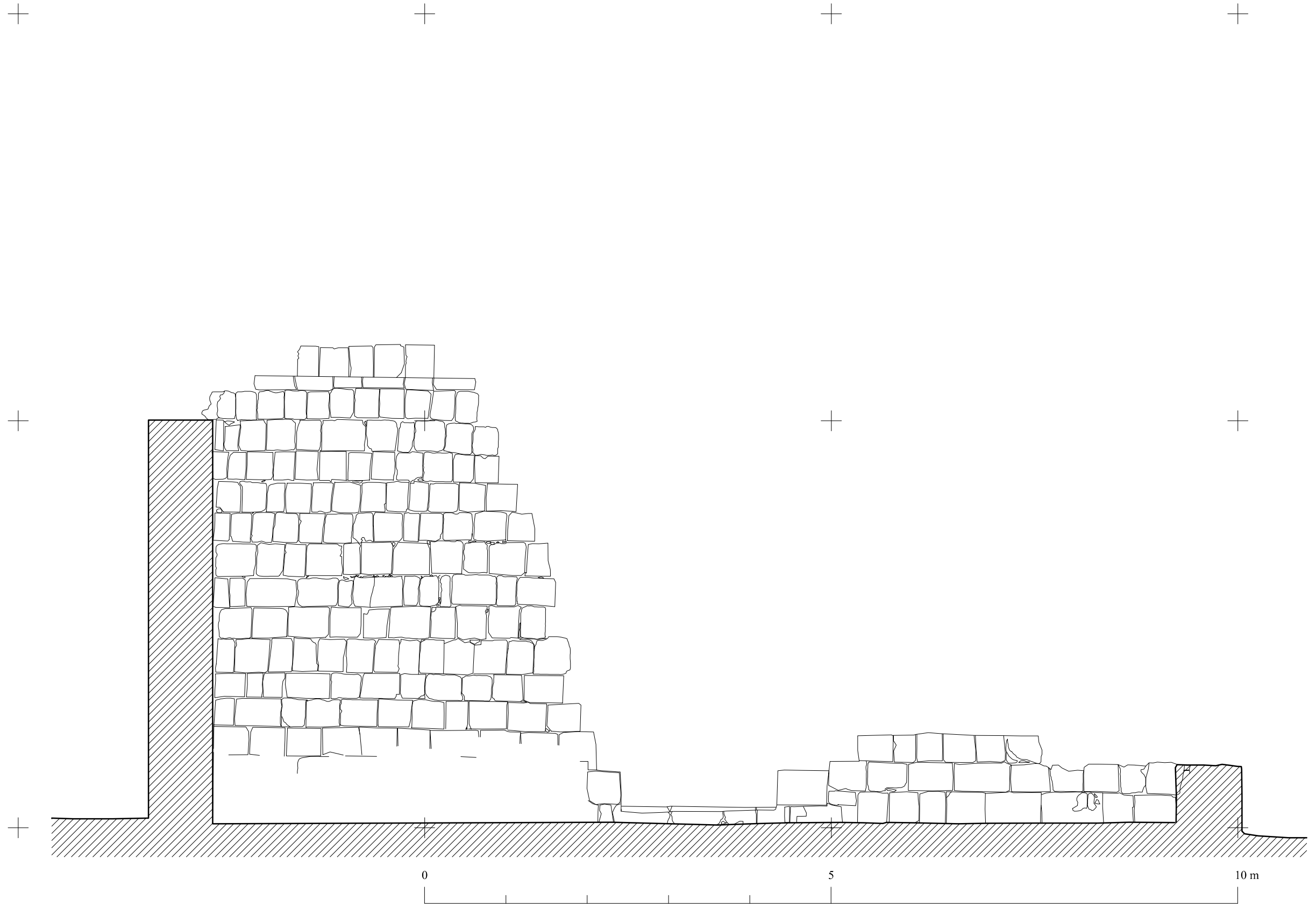
MEZQUITA DE QASR AL-HALLABAT. ALZADO INTERIOR NORTE. A. ALMAGRO / arq. MISION ARQUEOLOGICA ESPAÑOLA EN JORDANIA. NOV. 1.989
