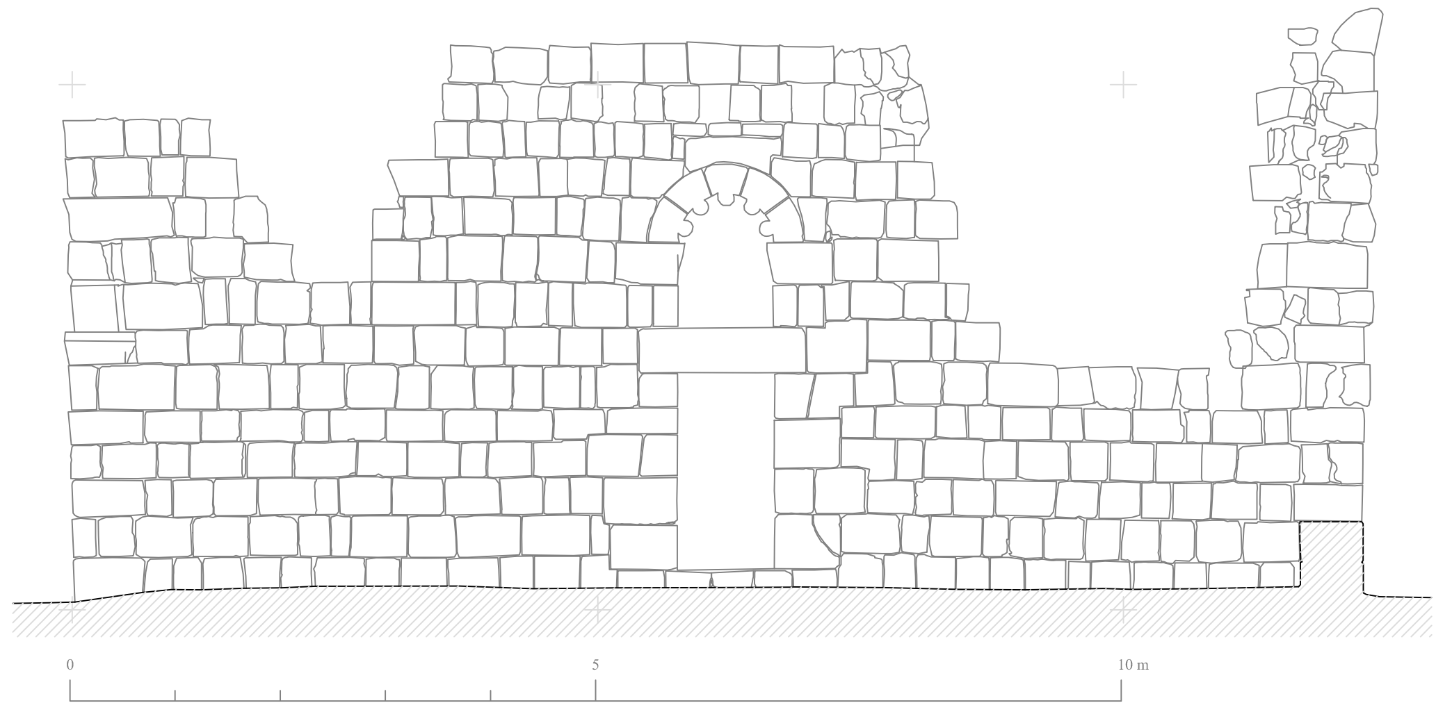
MEZQUITA DE QASR AL-HALLABAT. ALZADO EXTERIOR OESTE.
