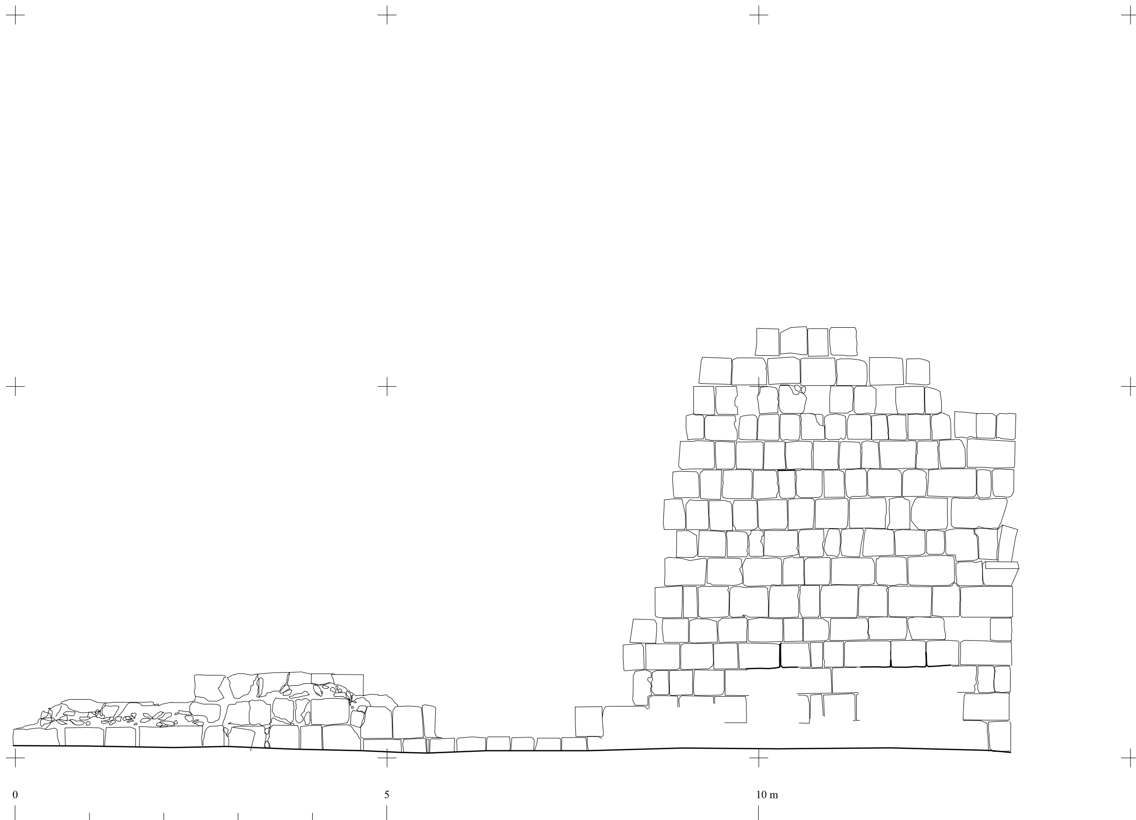
MEZQUITA DE QASR AL-HALLABAT. ALZADO EXTERIOR NORTE.
