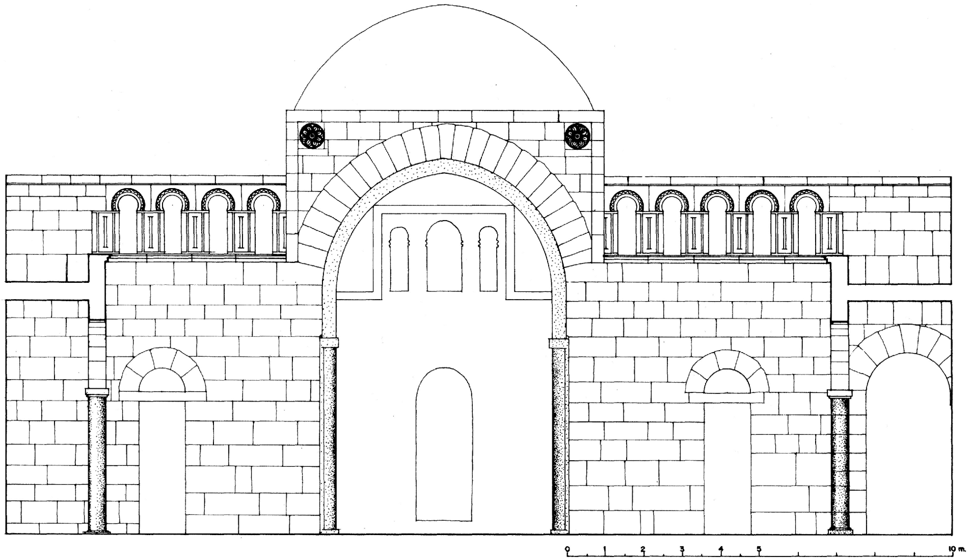
ALZADO DEL IWAN. HIPOTESIS
