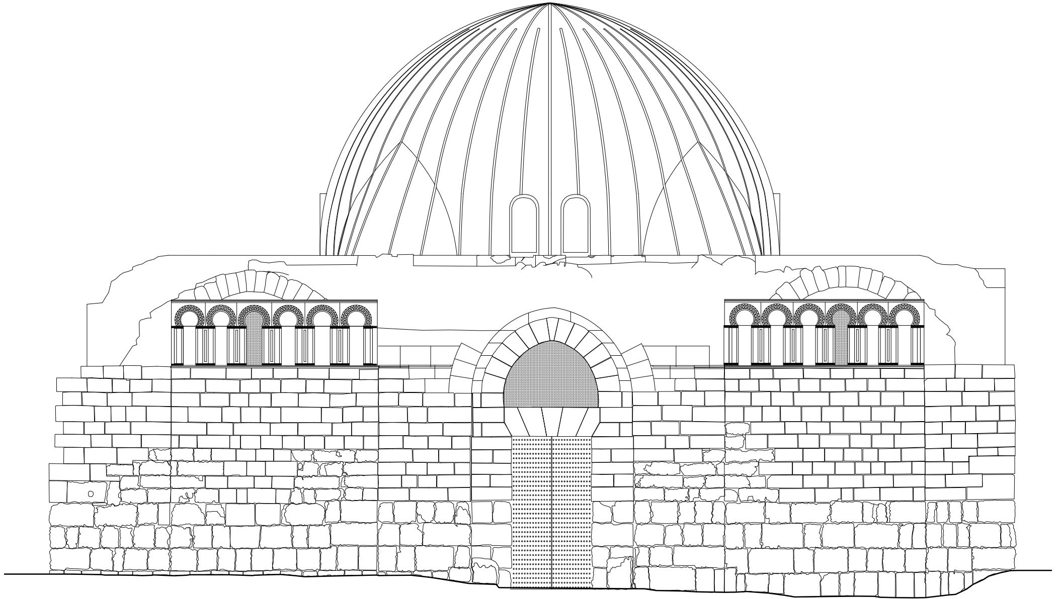
PALACIO OMEYA DE AMMAN. VESTIBULO. ALZADO SUR.
