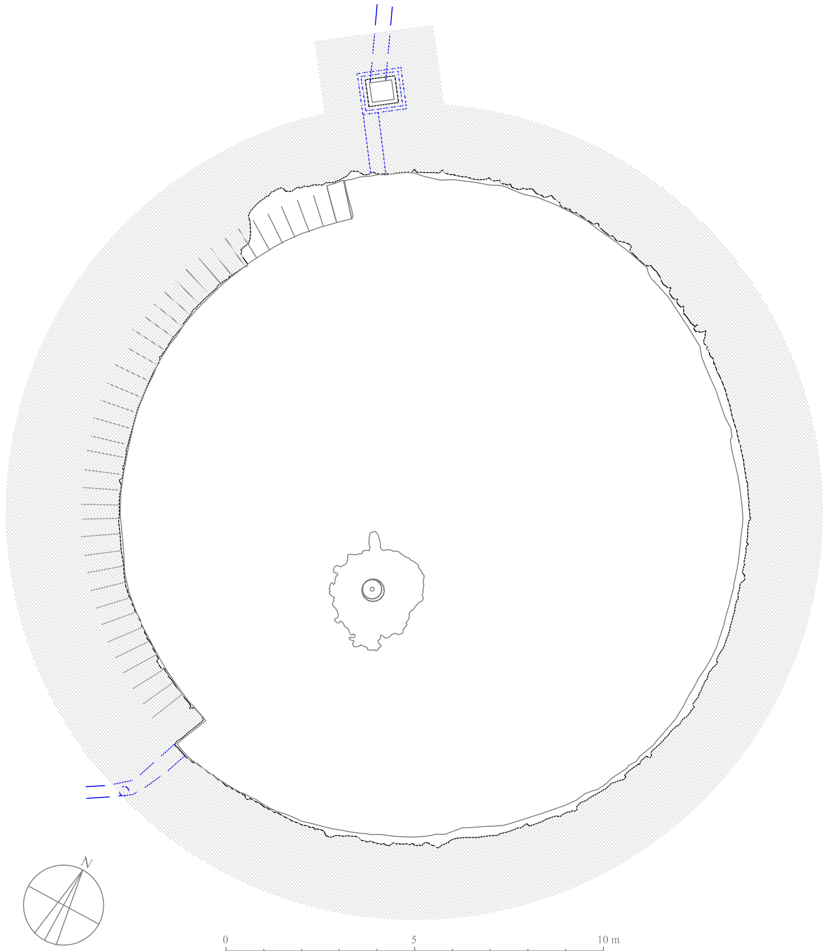
PALACIO OMEYA DE AMMAN. ALBERCÓN CIRCULAR. ESCUELA DE ESTUDIOS ARABES. A.ALMAGRO/arq. PLANTA.
