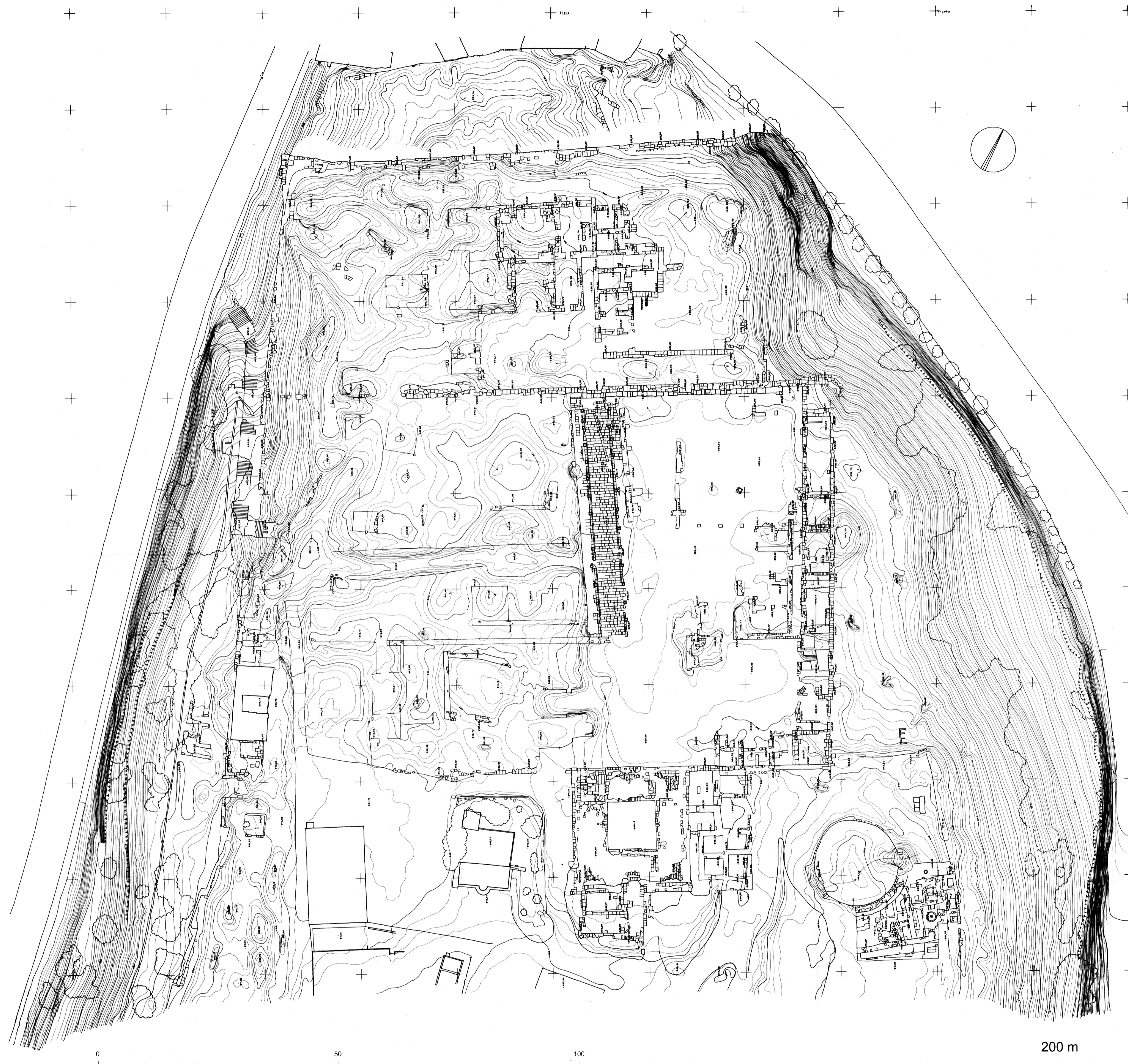
CIUDADELA DE AMMAN. JORDANIA. PLANTA DEL AREA DEL ALCÁZAR
