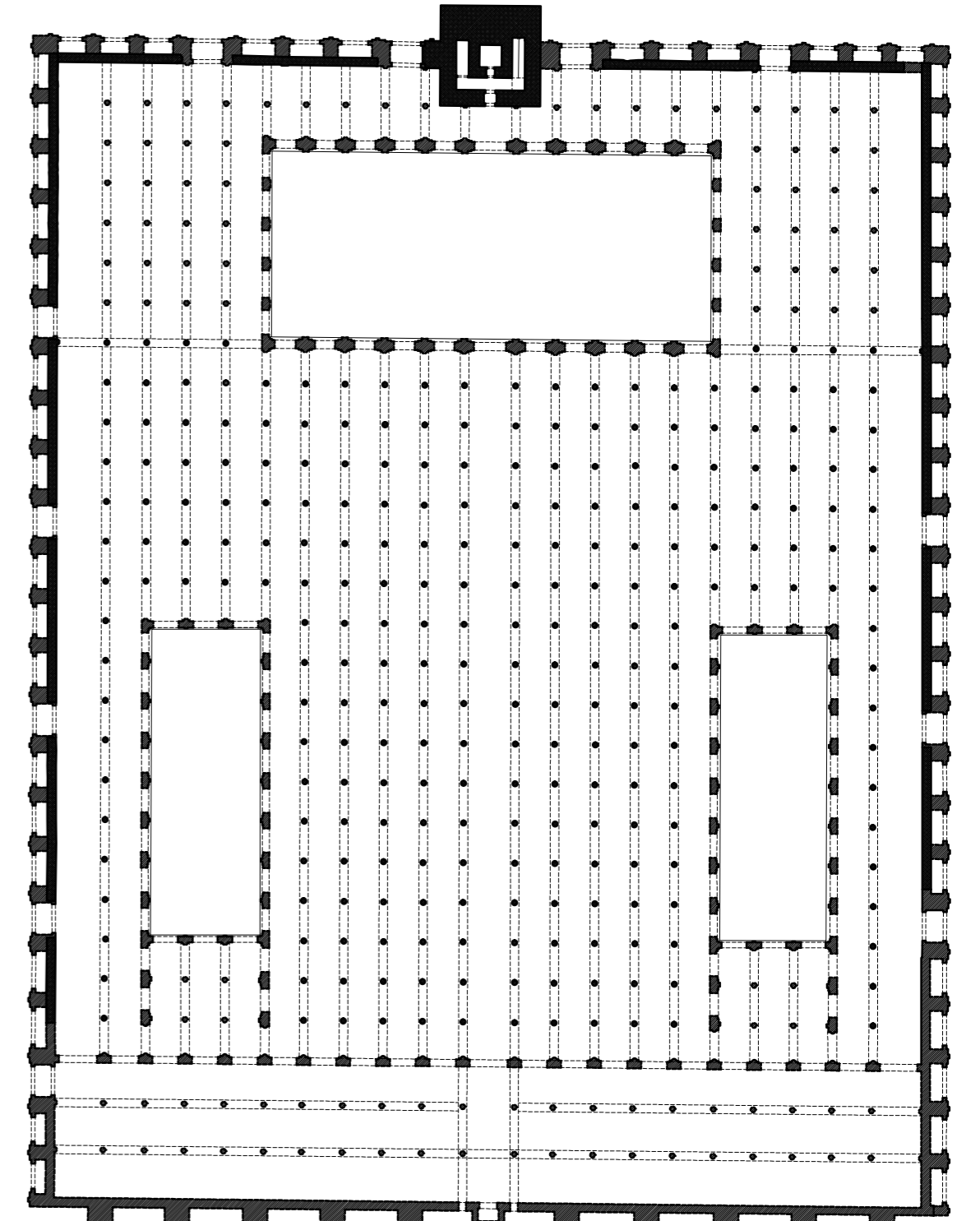
MEZQUITA ALMOHADE DE RABAT. PLANTA. ESCUELA DE ESTUDIOS ARABES, C.S.I.C. ALMAGRO yS.
