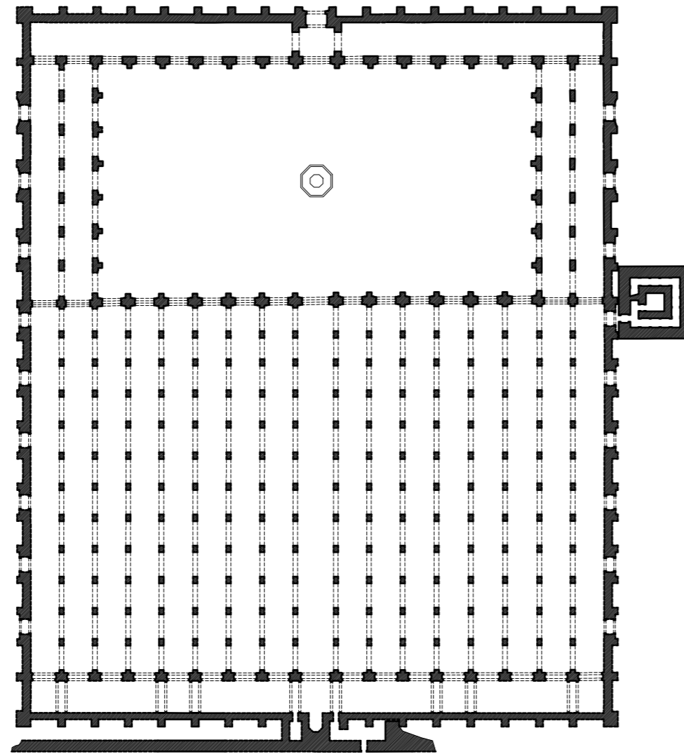
MEZQUITA ALMOHADE DE SEVILLA. PLANTA. ESCUELA DE ESTUDIOS ARABES, C.S.I.C. ALMAGRO yS. ALJENECI yS.
