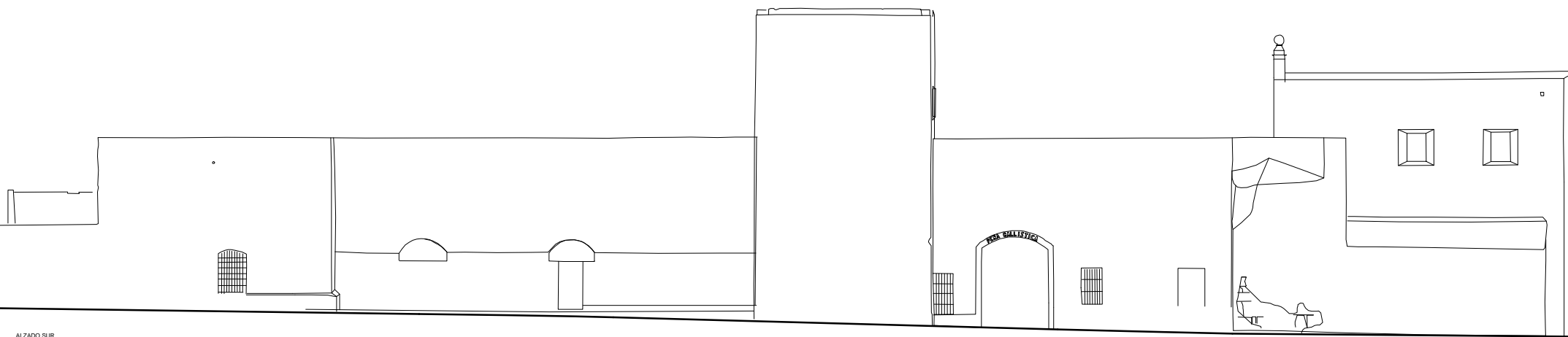
ALZADO SUR
