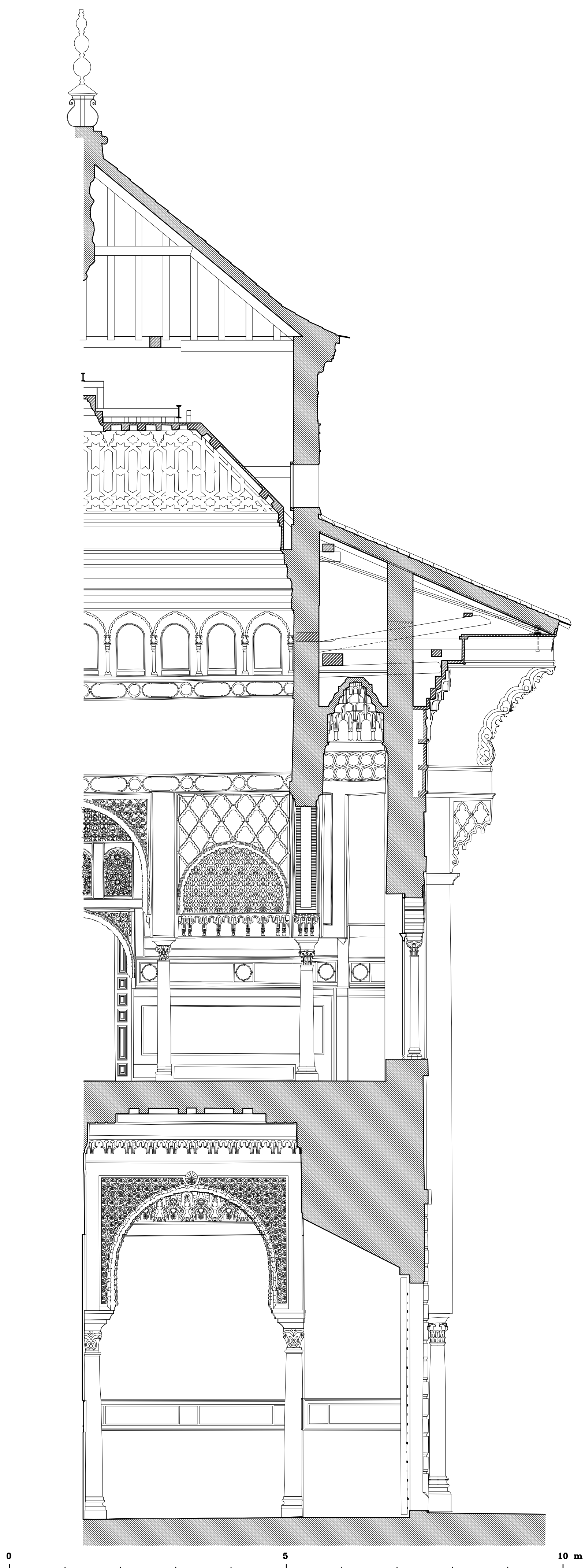
PALACIO DE PEDRO I EN EL ALCAZAR DE SEVILLA. SECCION DE LA PORTADA Y EL ALERO
