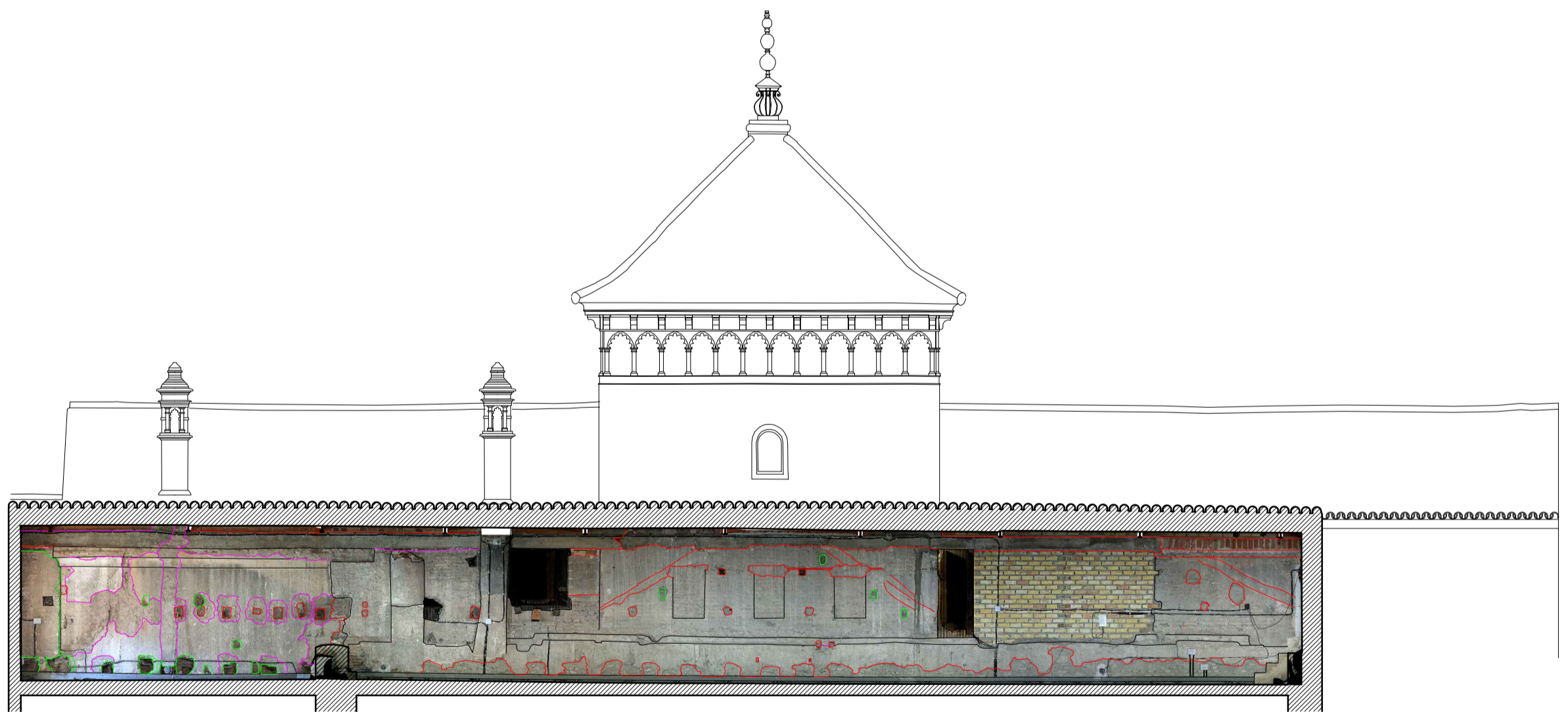
ALCAZAR DE SEVILLA. PALACIO DE PEDRO I. PLANTA Y ALZADO DEL CAMARANCHÓN BAJO EL TEJADO DE LAS CRUJÍAS SEPTENTRIONALES DEL PALACIO Escuela de Estudios Árabes, CSIC, Antonio Almagro / arquitecto noviembre 2015
