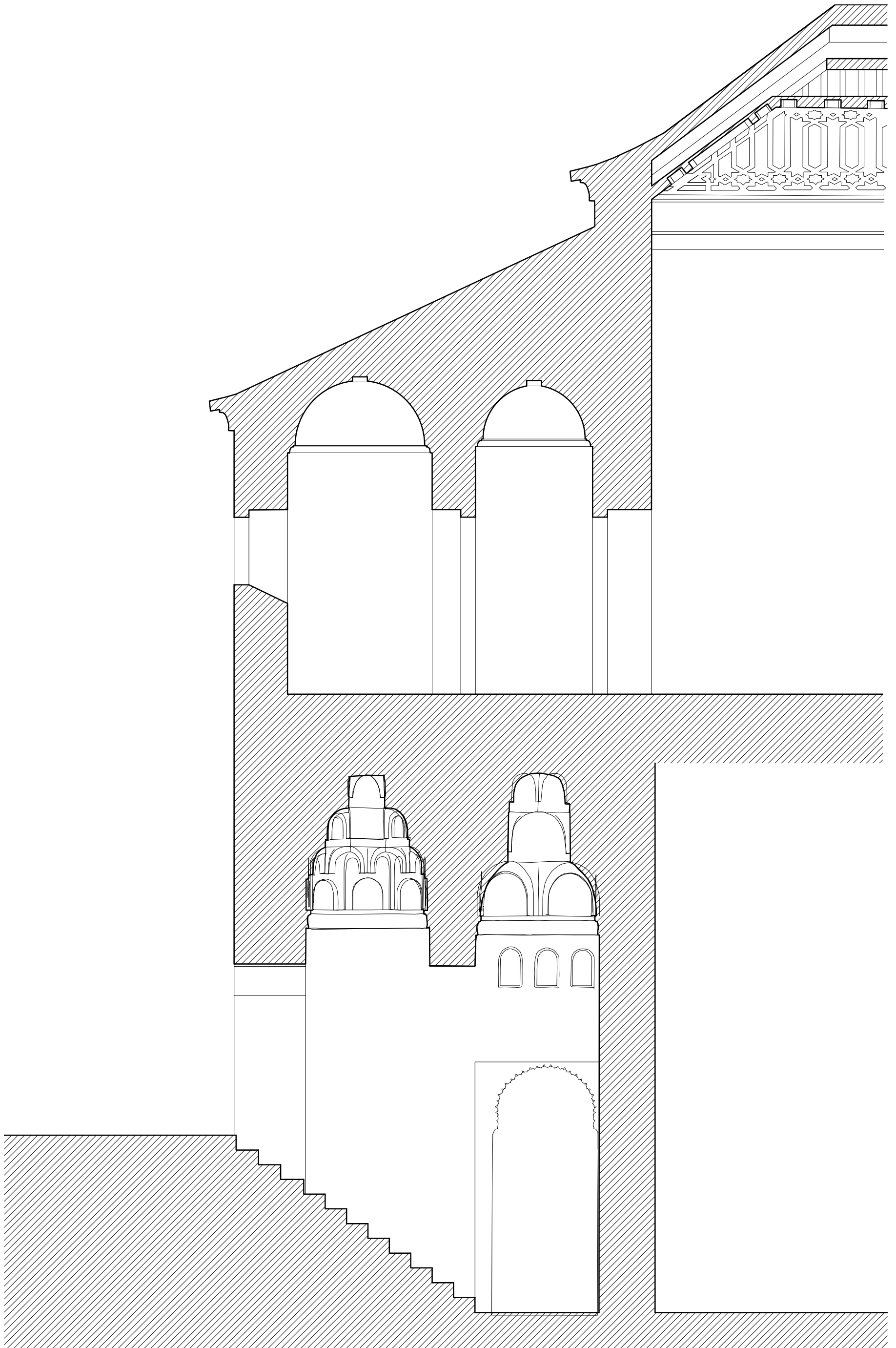
0 1 2 3 m ALCAZAR DE SEVILLA. PALACIO DE PEDRO I ACCESO AL PATIO DE LAS DONCELLAS A.ALMAGRO/ARQ. ESCUELA DE ESTUDIOS ARABES C.S.I.C.
