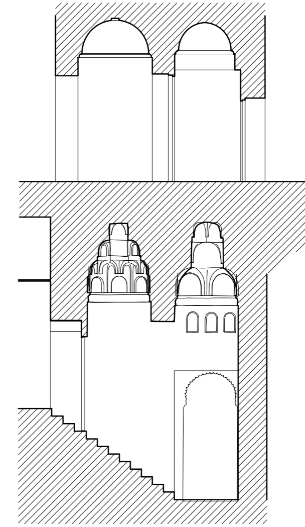
SECCION F
