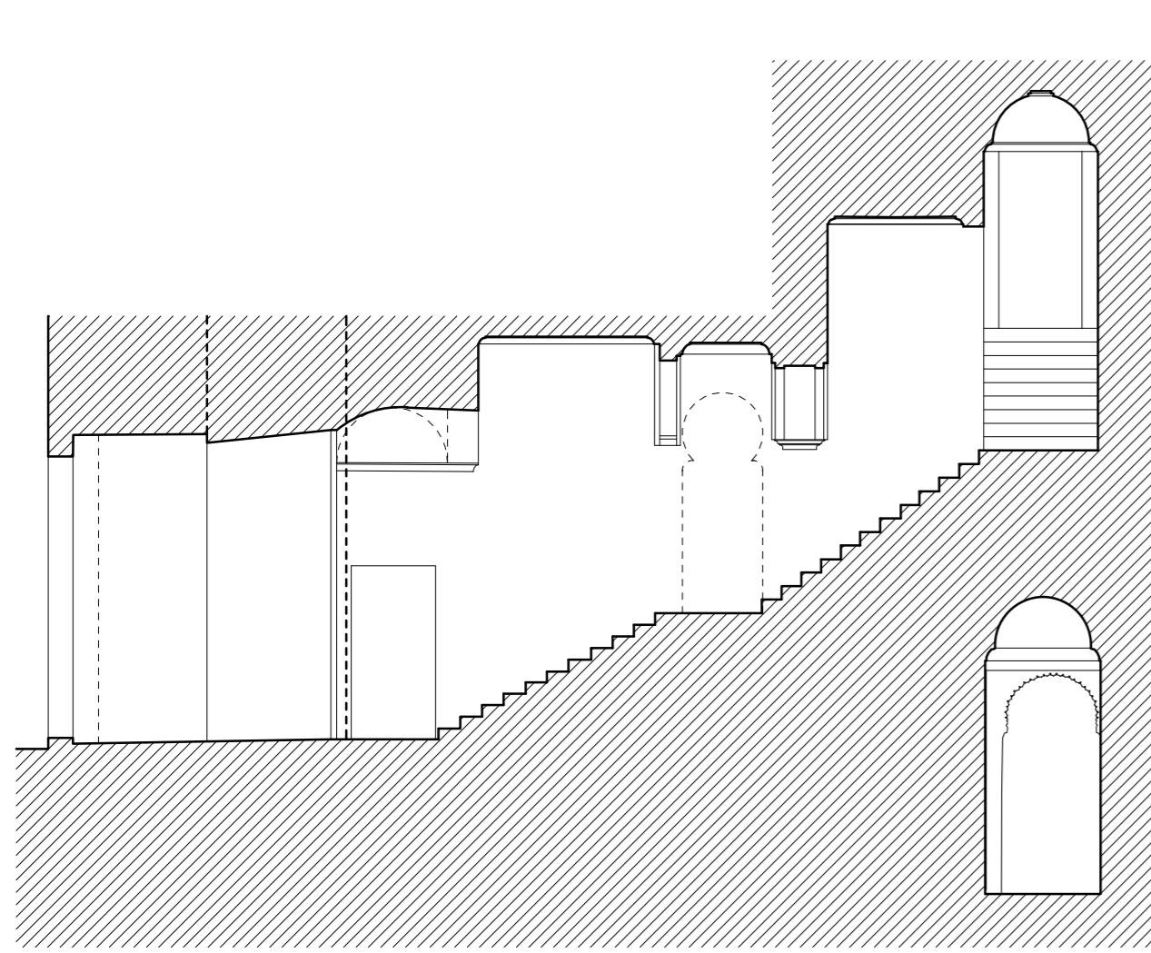
SECCION C
