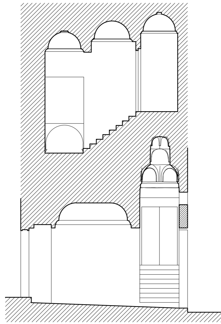
SECCION D
