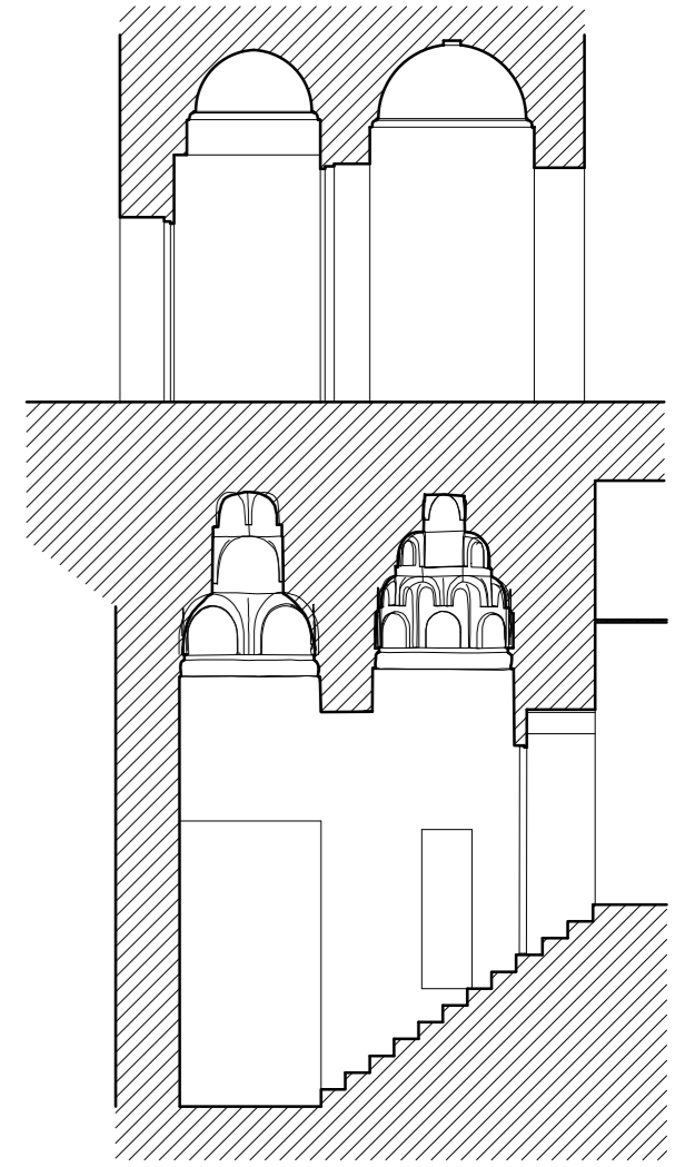
SECCION G
