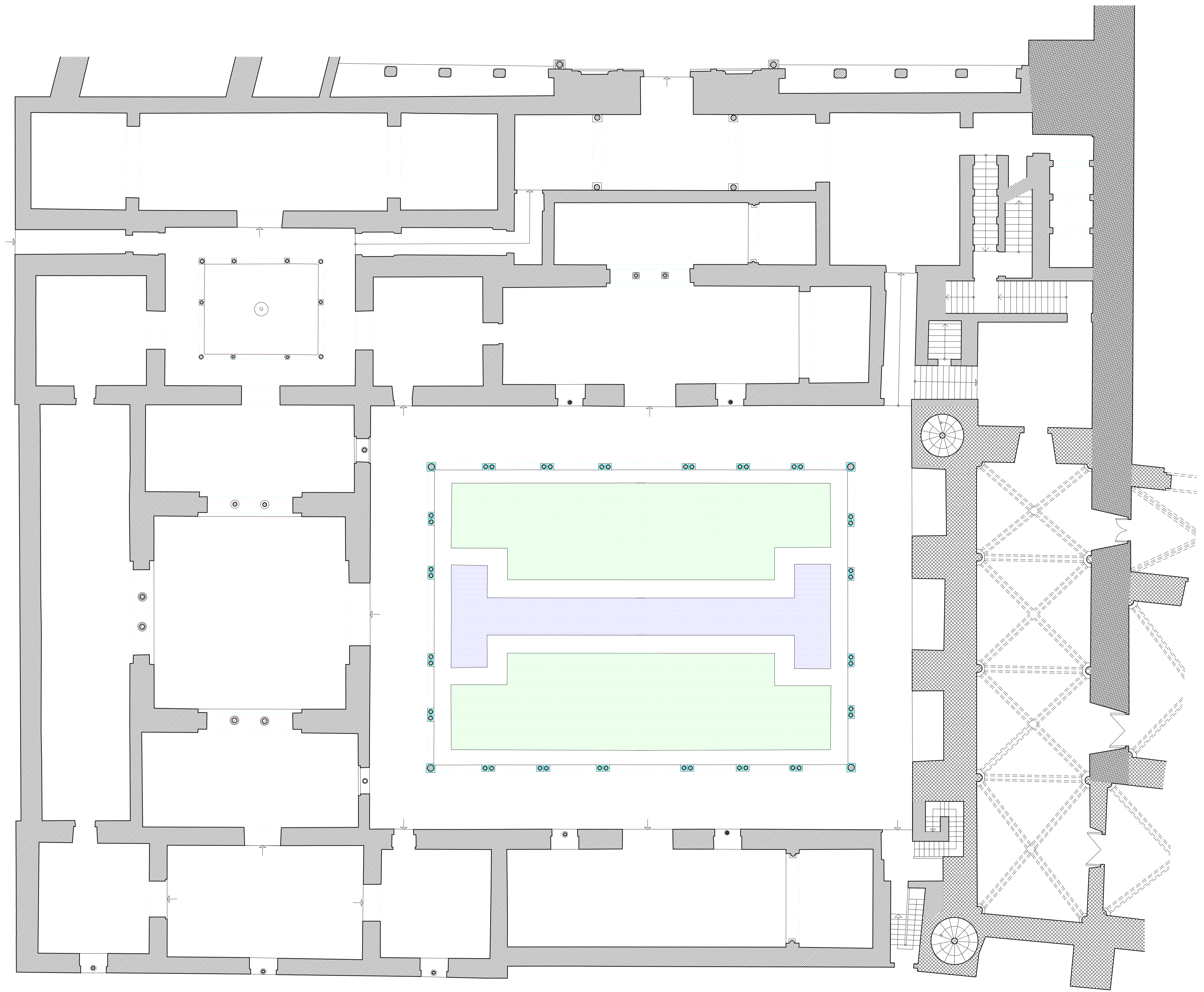
REALES ALCAZARES DE SEVILLA. PALACIO MUDEJAR DEL REY PEDRO I. HIPOTESIS DE PLANTA BAJA. ESCUELA DE ESTUDIOS ARABES, C.S.I.C. A. ALMAGRO o arq.
