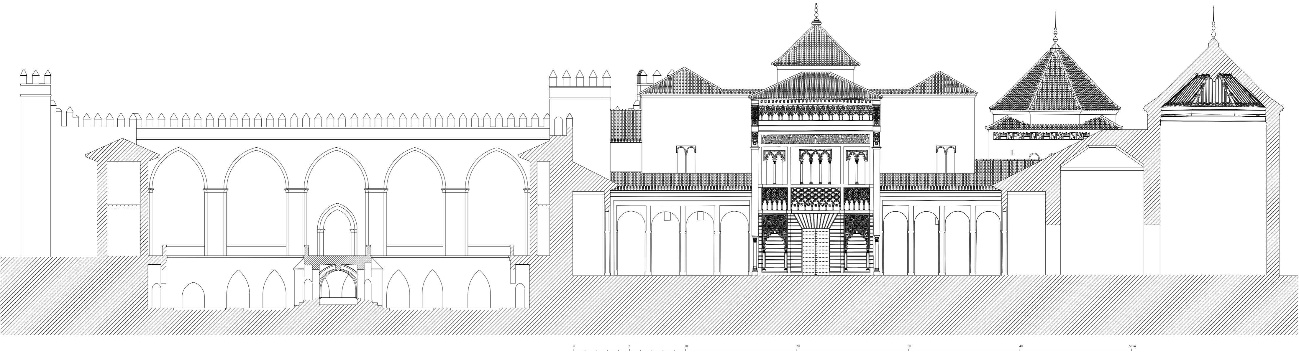
REALES ALCAZARES DE SEVILLA. PALACIO DEL REY PEDRO I. HIPOTESIS DE FACHADA. ESCUELA DE ESTUDIOS ARABES. C.S.I.C. A. ALMAGRO arq.
