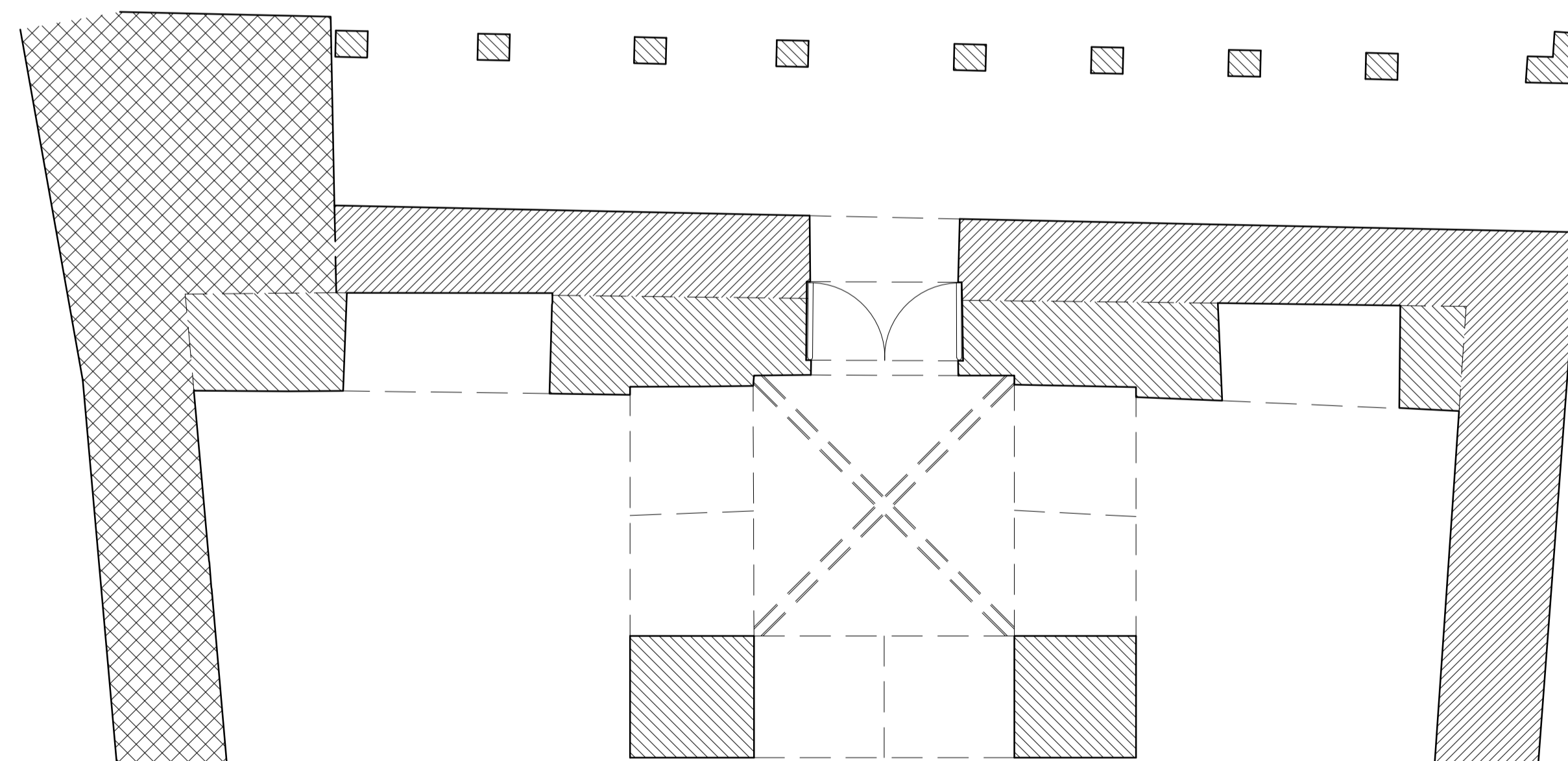
ALCAZAR DE SEVILLA. PUERTA DE LA MONTERIA. DISEÑO DE REPOSICION ALABR. C. 111. G. LAMARCA/ 89.
