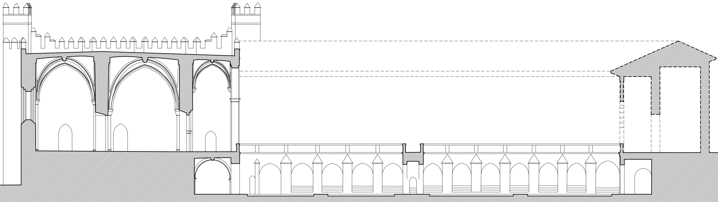
ALCAZAR DE SEVILLA. PATIO DEL CRUCERO. HIPOTESIS DEL PATIO GOTICO. ESCUELA DE ESTUDIOS ARABES, C.S.I.C. A. ALMAGRO/ arq.
