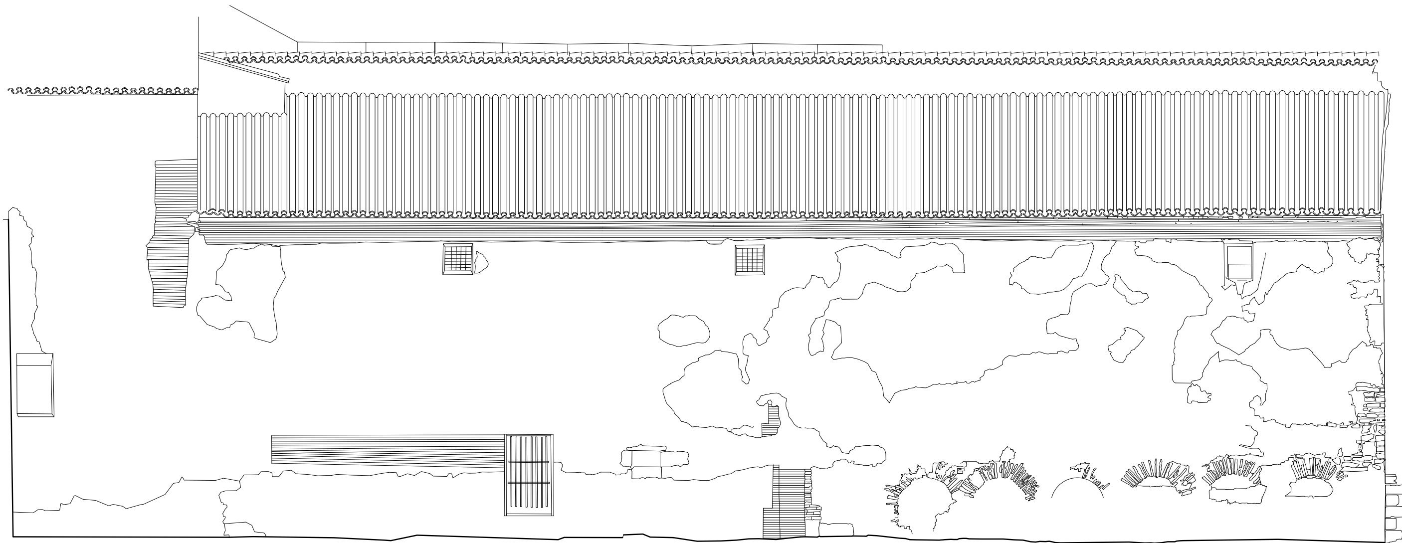
CONVENTO DE SANTA CLARA. TORDESILLAS. SALON DEL ALJIBE. ALZADO ESTE.
