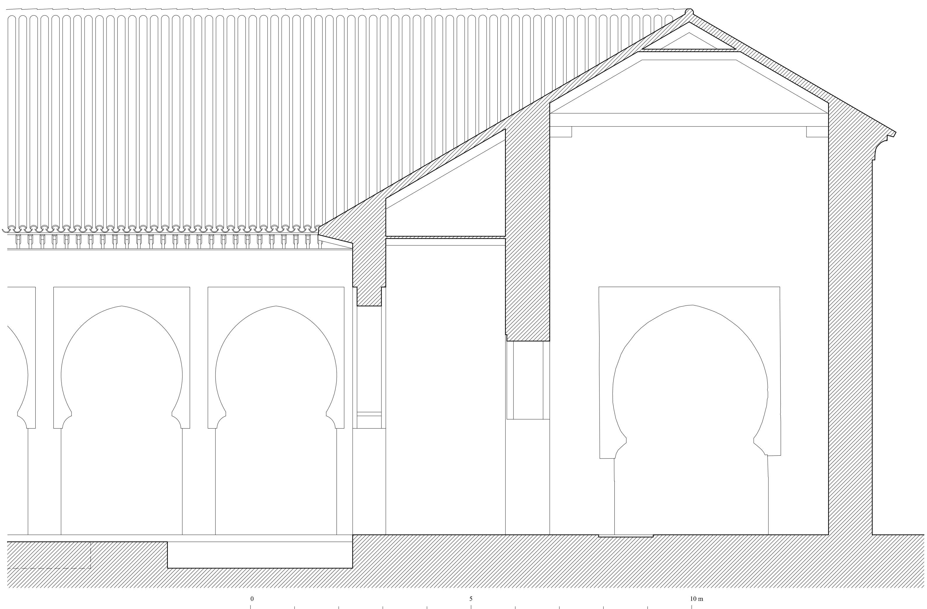
PALACIO DE PEDRO I EN TORDESILLAS. SALON DEL ALJIBE. SECCION HIPÓTESIS.
