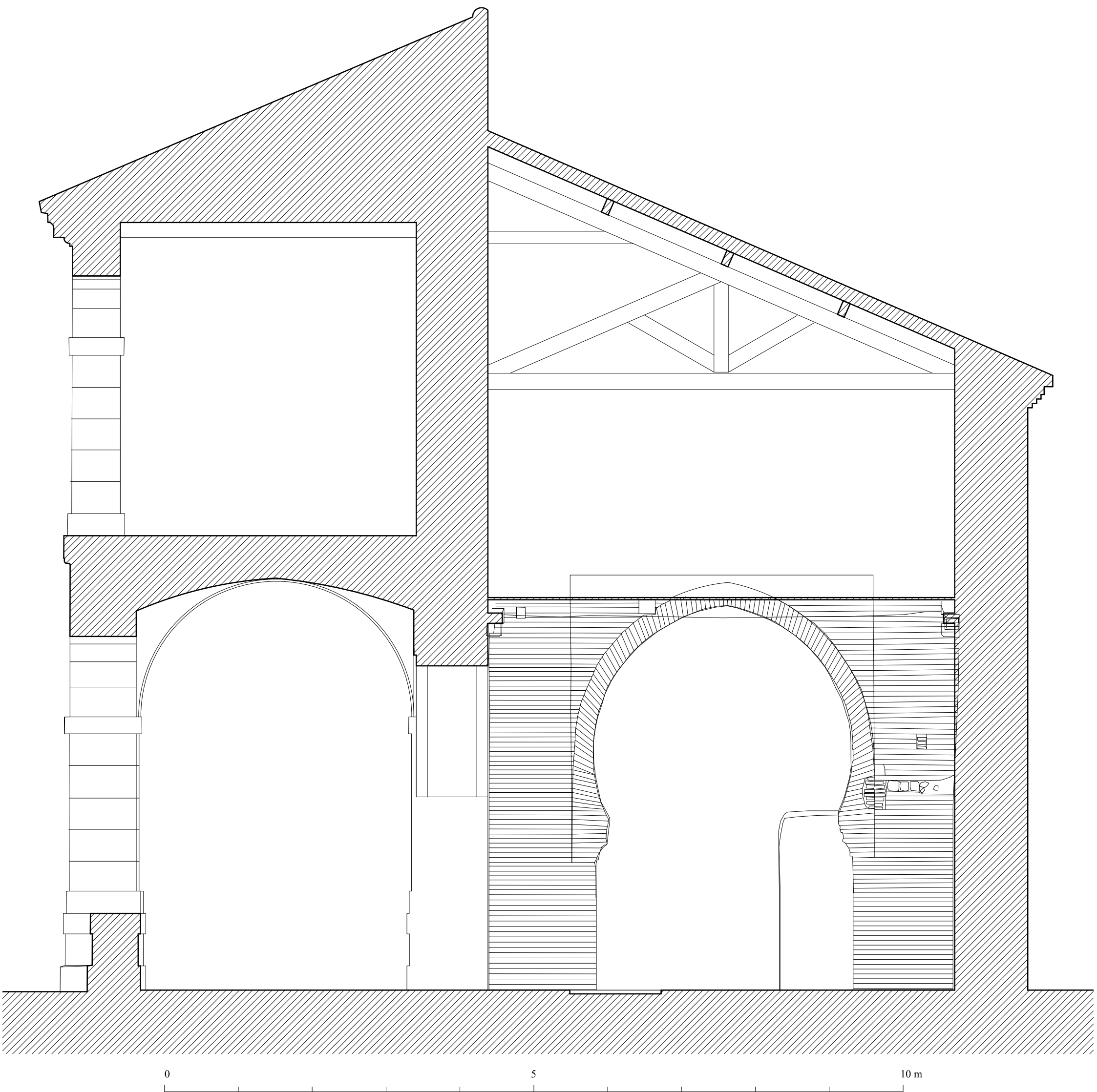
CONVENTO DE SANTA CLARA. TORDESILLAS. SALON DEL ALJIBE. SECCION.
