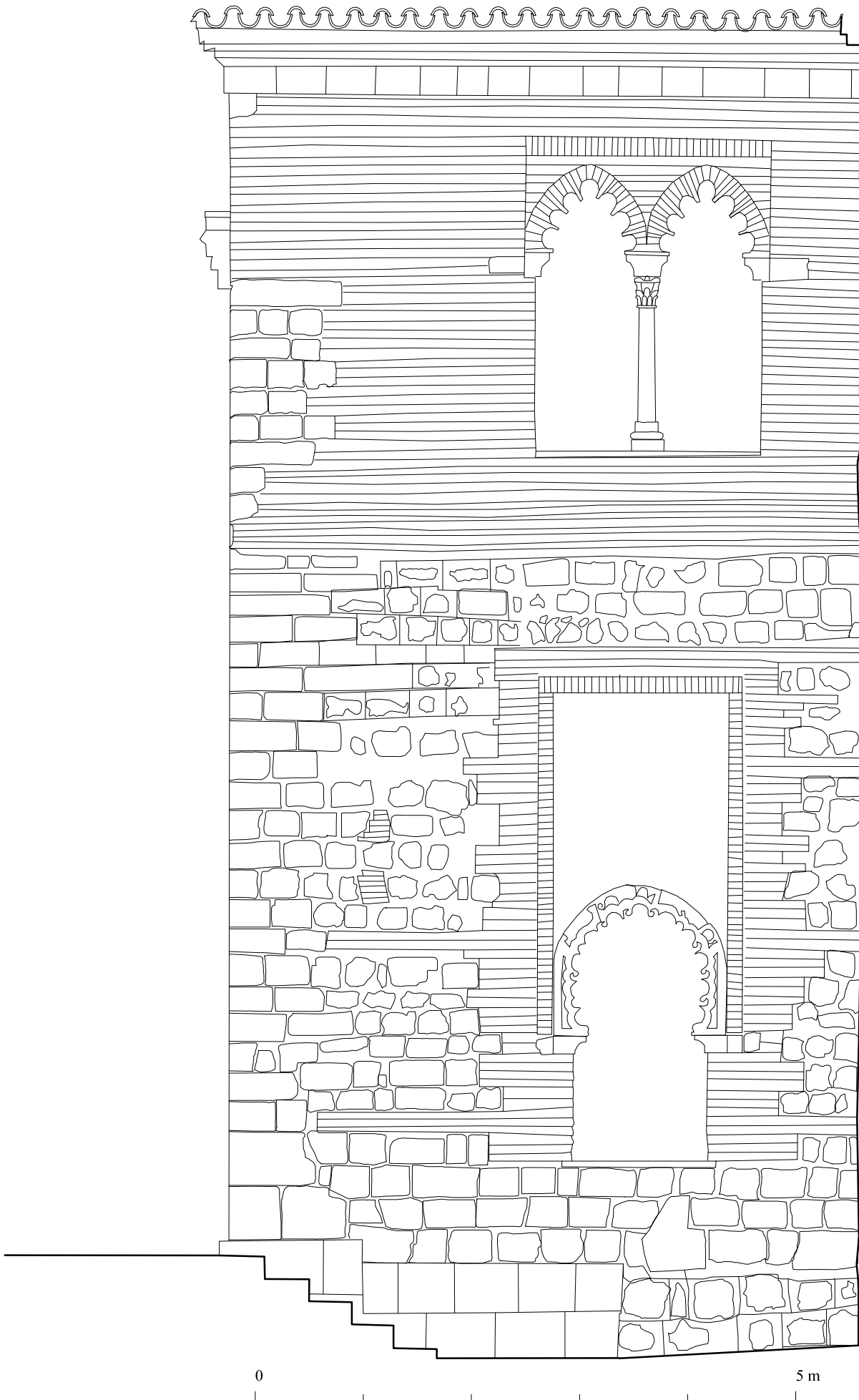
CONVENTO DE SANTA CLARA. TORDESILLAS. PUERTA DEL PALACIO. ALZADO SUR.
