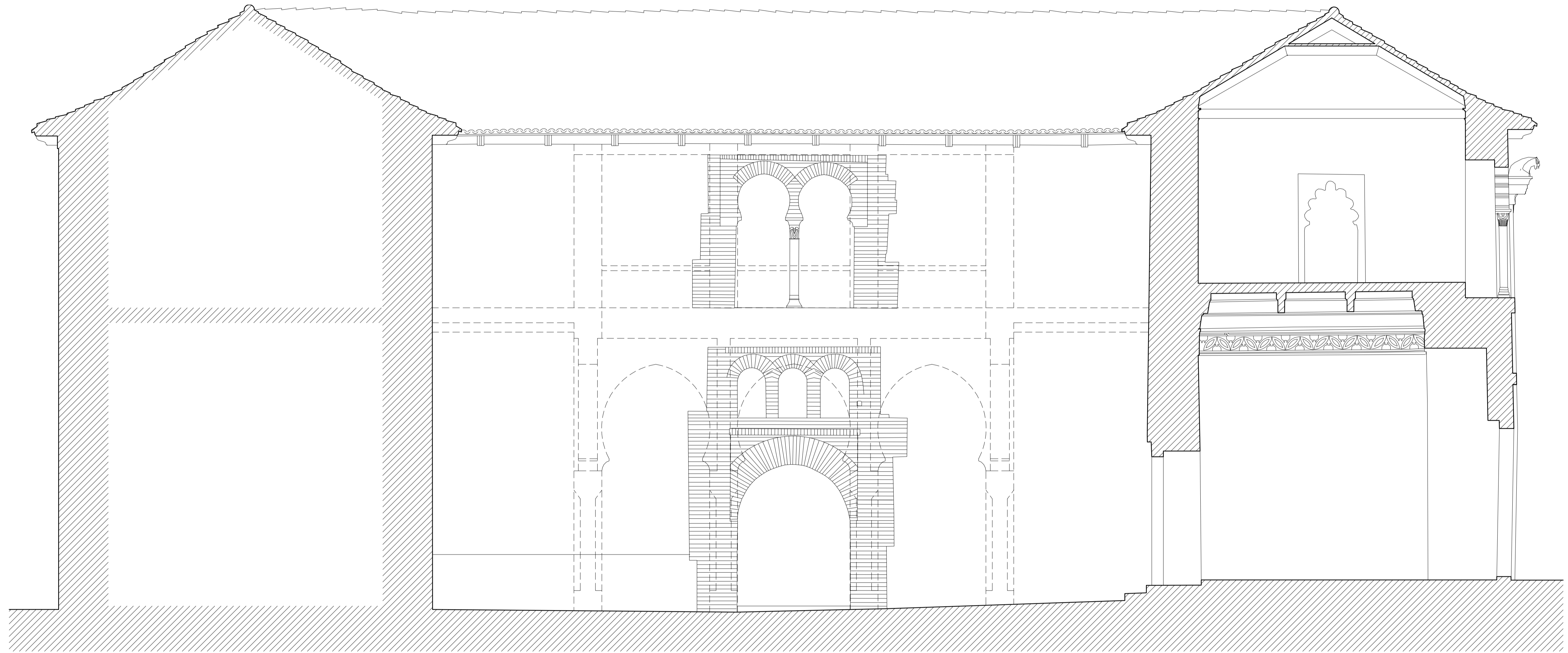
PALACIO DE ASTUDILLO SECCIÓN DEL PATIO Y EL VESTÍBULO ESCUELA DE ESTUDIOS ARABES, C.S.I.C. A. Almagro/ arq.
