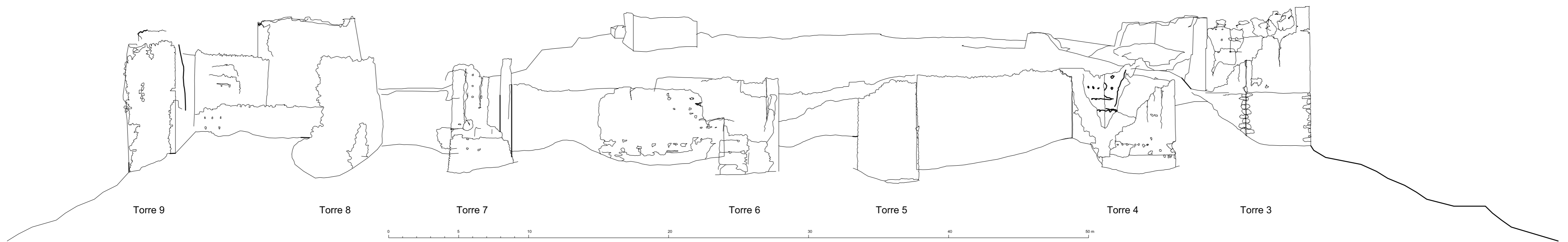
CASTILLO DE PIÑAR (GRANADA).ALZADO SUR. A. Almagro/arq. Escuela de Estudios Arabes, CSIC
