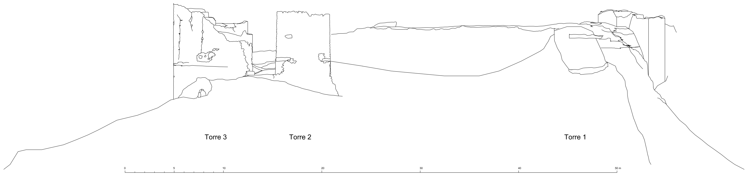
CASTILLO DE PIÑAR (GRANADA). ALZADO NORTE.
