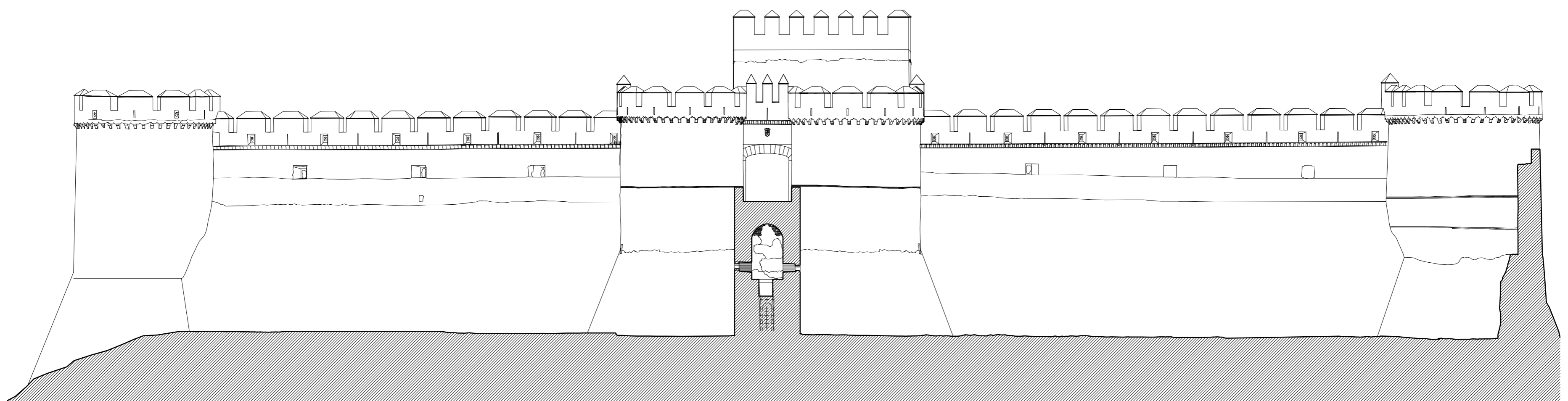
CASTILLO DE SAN MIGUEL (ALMUÑÉCAR) BARRERA DE ARTILLERÍA DEL LADO NORTE (SIGLO XV-XVI) ESCUELA DE ESTUDIOS ARABES (C.S.I.C.) A. ALMAGRO/ A. ORIHUELA, arqts.
