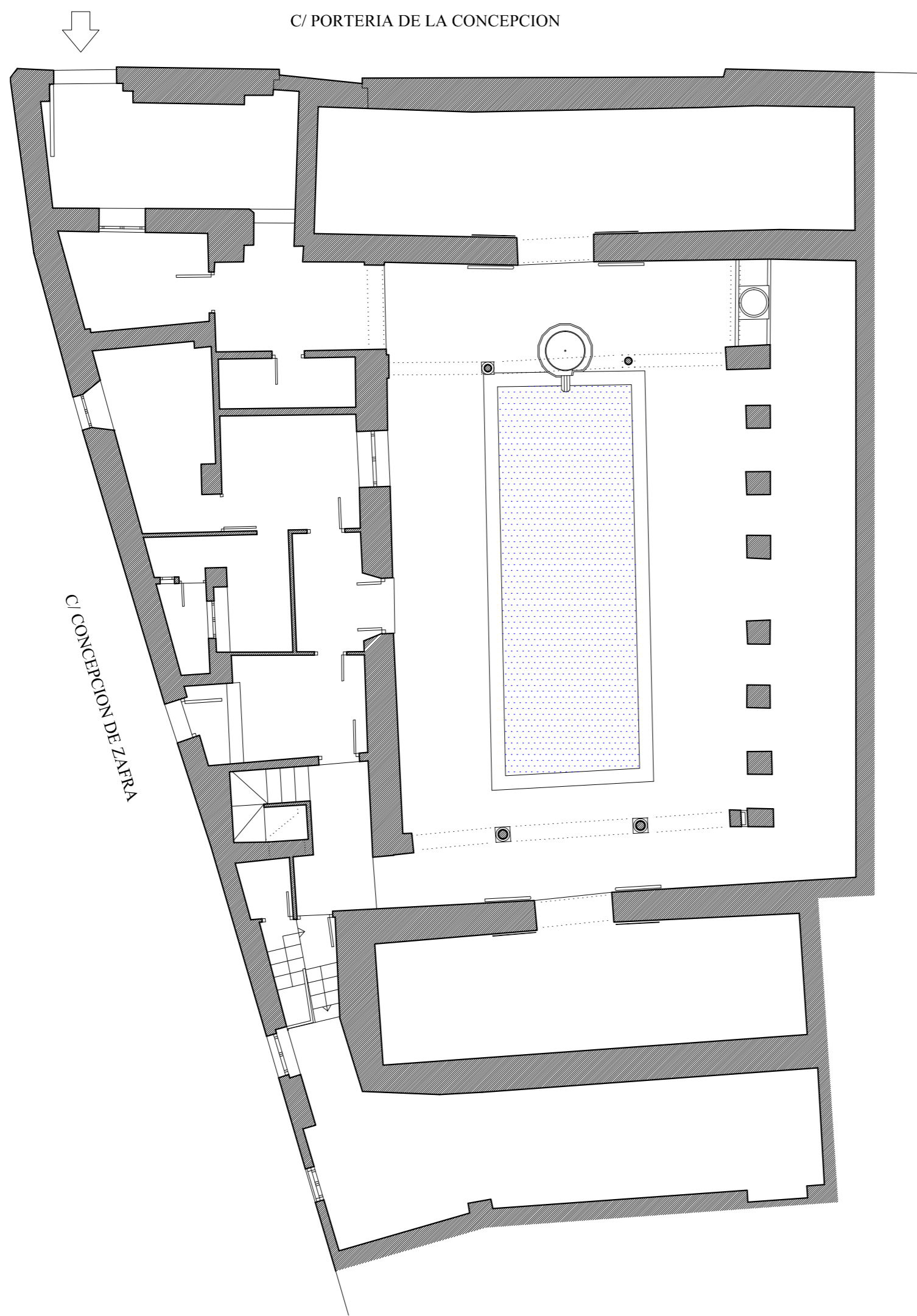
PLANTA BAJA
