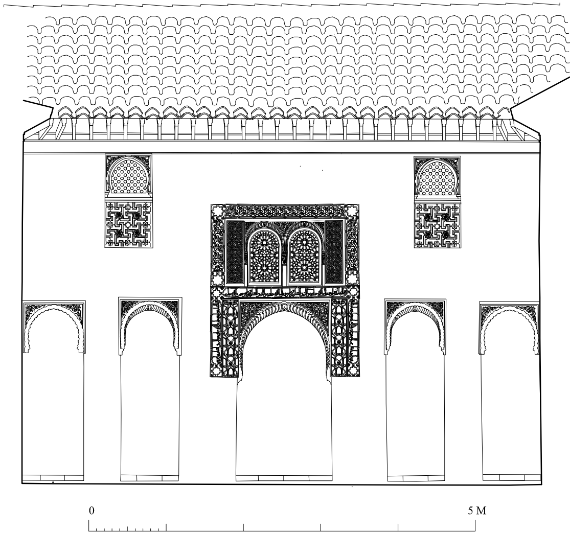
CASA EN C/COBERTIZO DE SANTA INES. GRANADA. SECCION HACIA SUR. HIPÓTESIS
