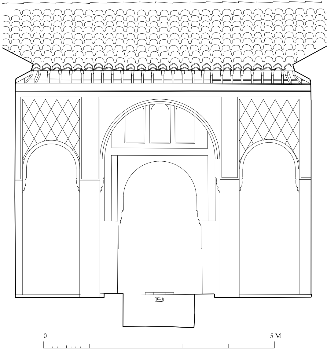
CASA EN C/COBERTIZO DE SANTA INES. GRANADA. SECCION HACIA NORTE. HIPÓTESIS
